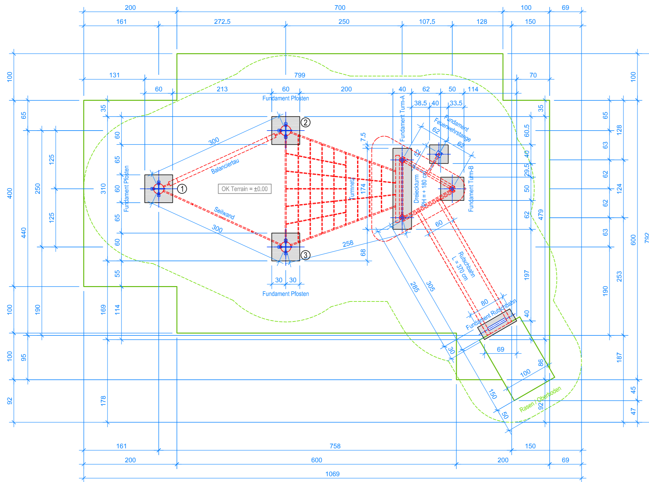
GRUNDRISS 1:50
