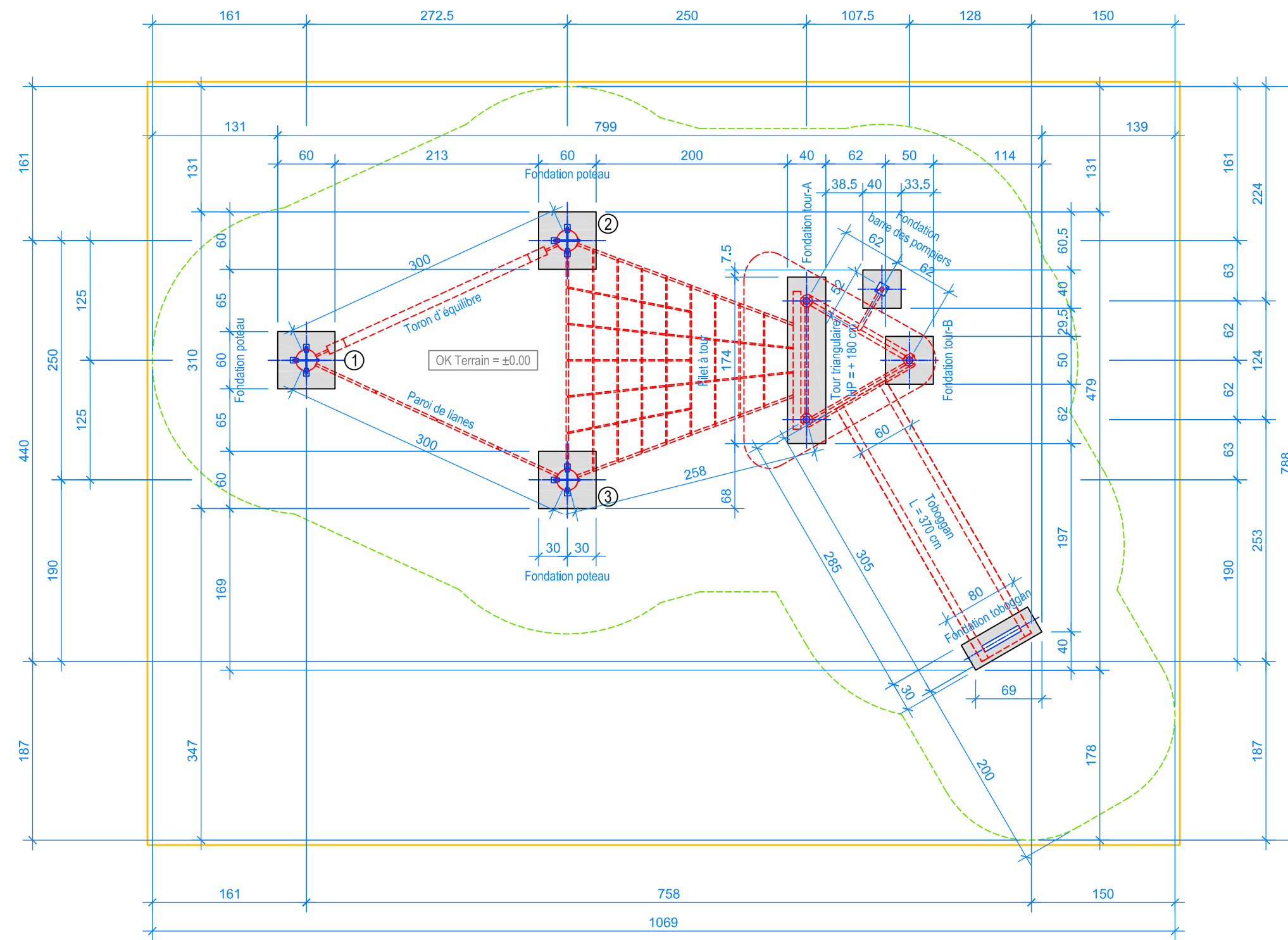
PLAN 1:50
