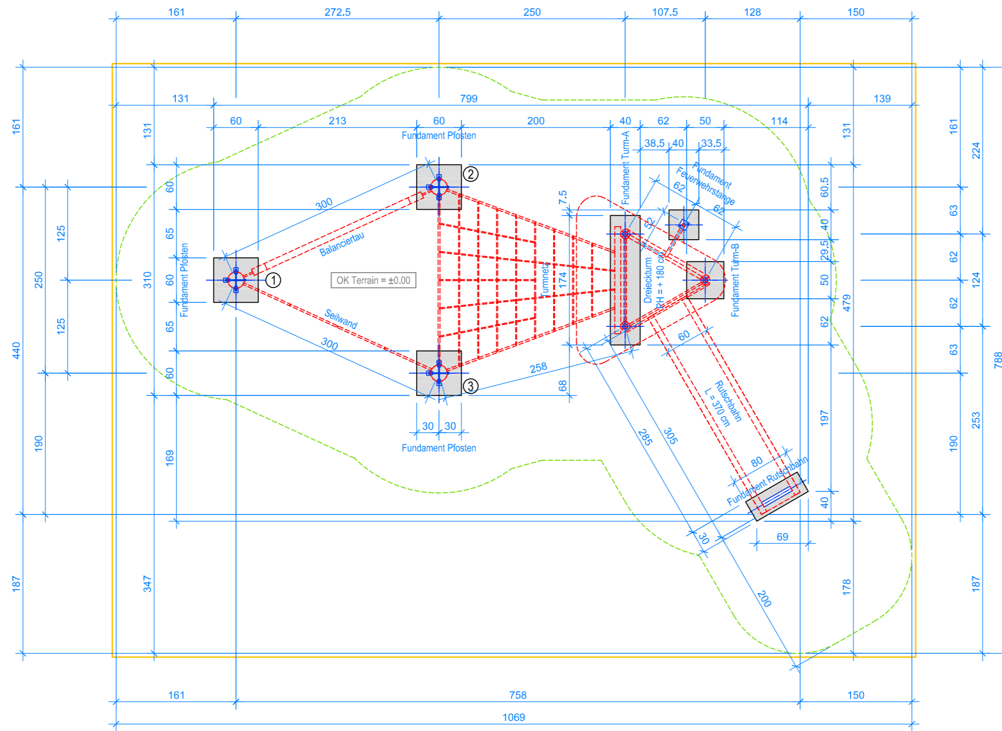
GRUNDRISS 1:50
