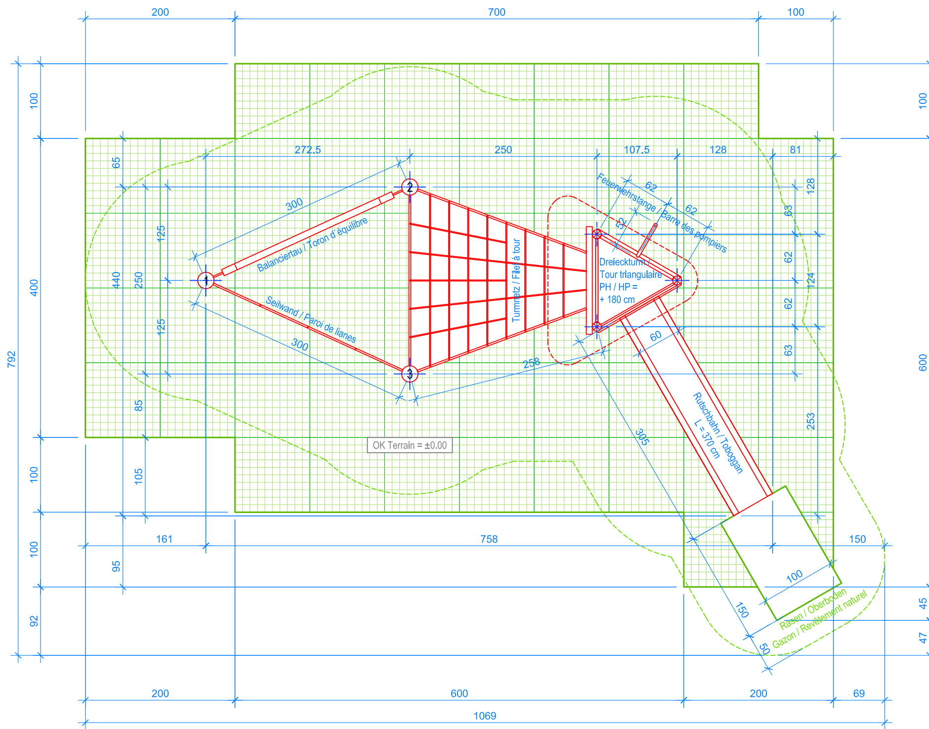
GRUNDRISS / PLAN 1:50
