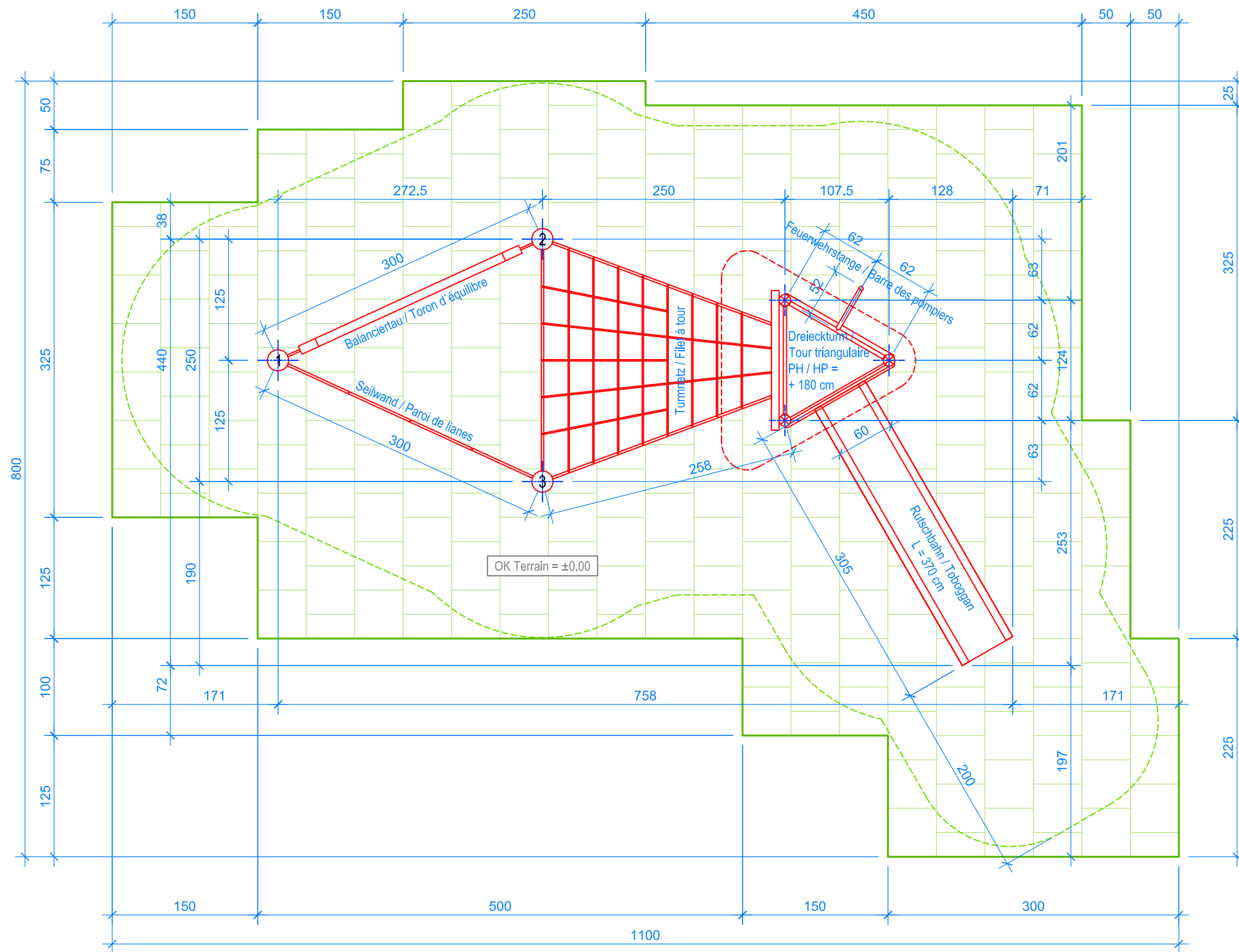
GRUNDRISS / PLAN 1:50
