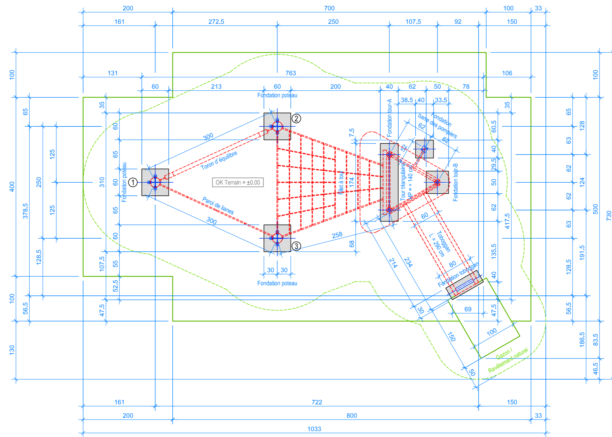
PLAN 1:50
