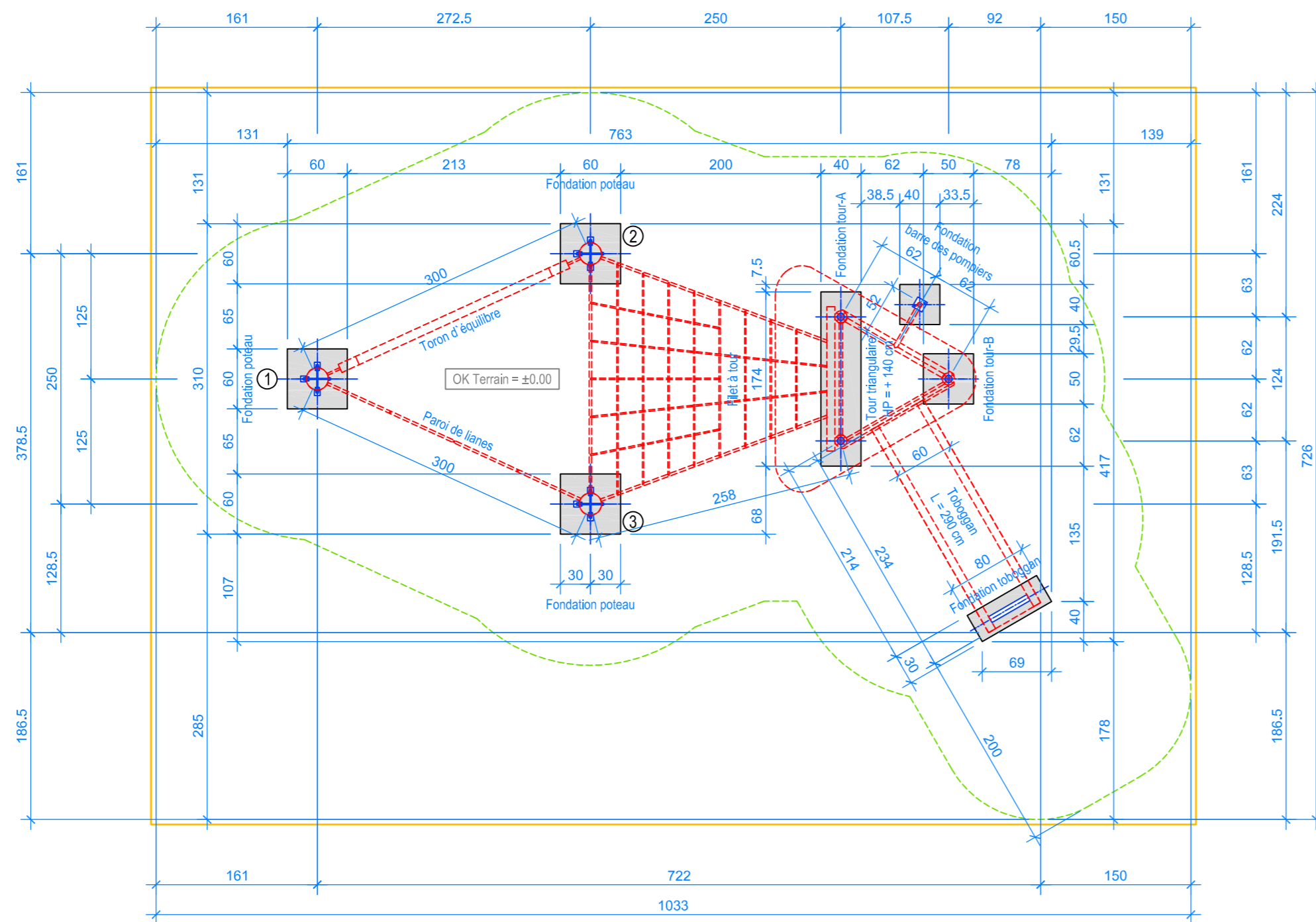
PLAN 1:50
