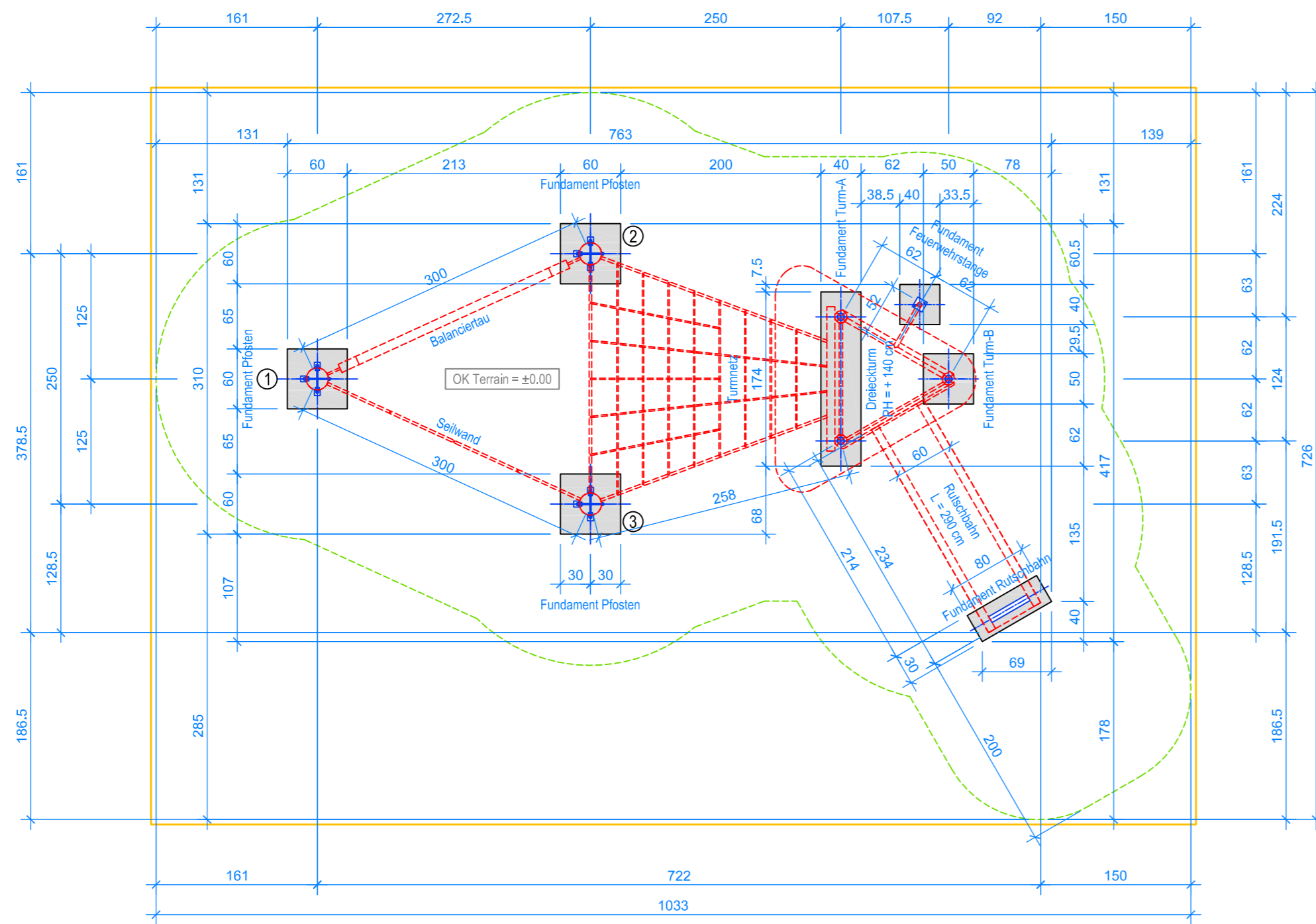
GRUNDRISS 1:50
