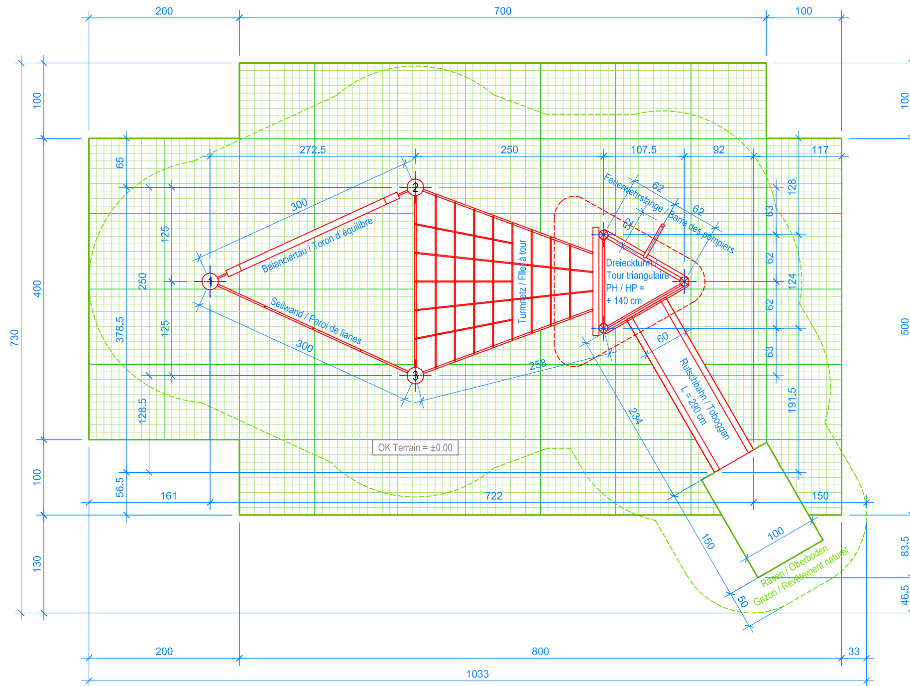
GRUNDRISS / PLAN 1:50
