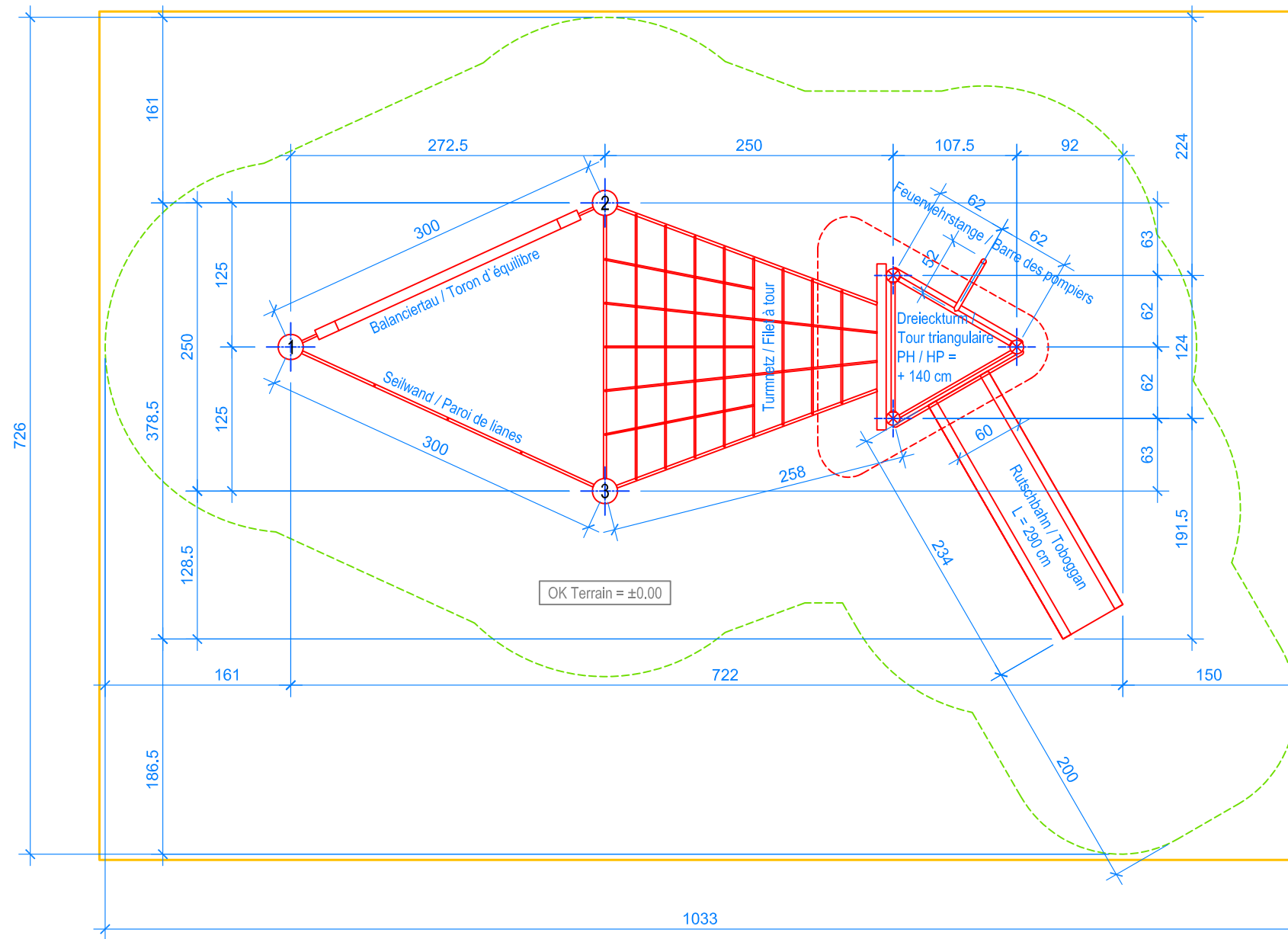
GRUNDRISS / PLAN 1:50
