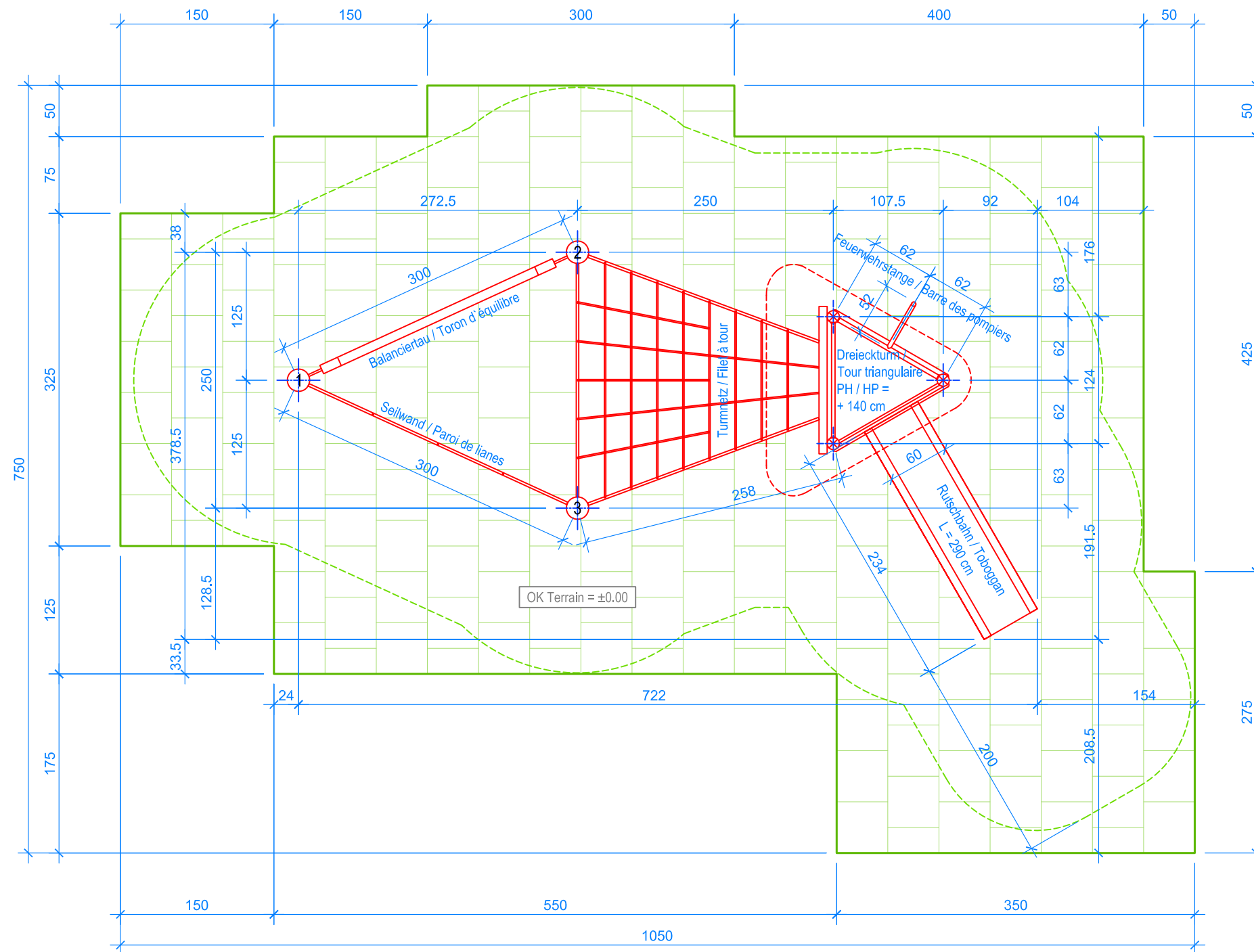
GRUNDRISS / PLAN 1:50
