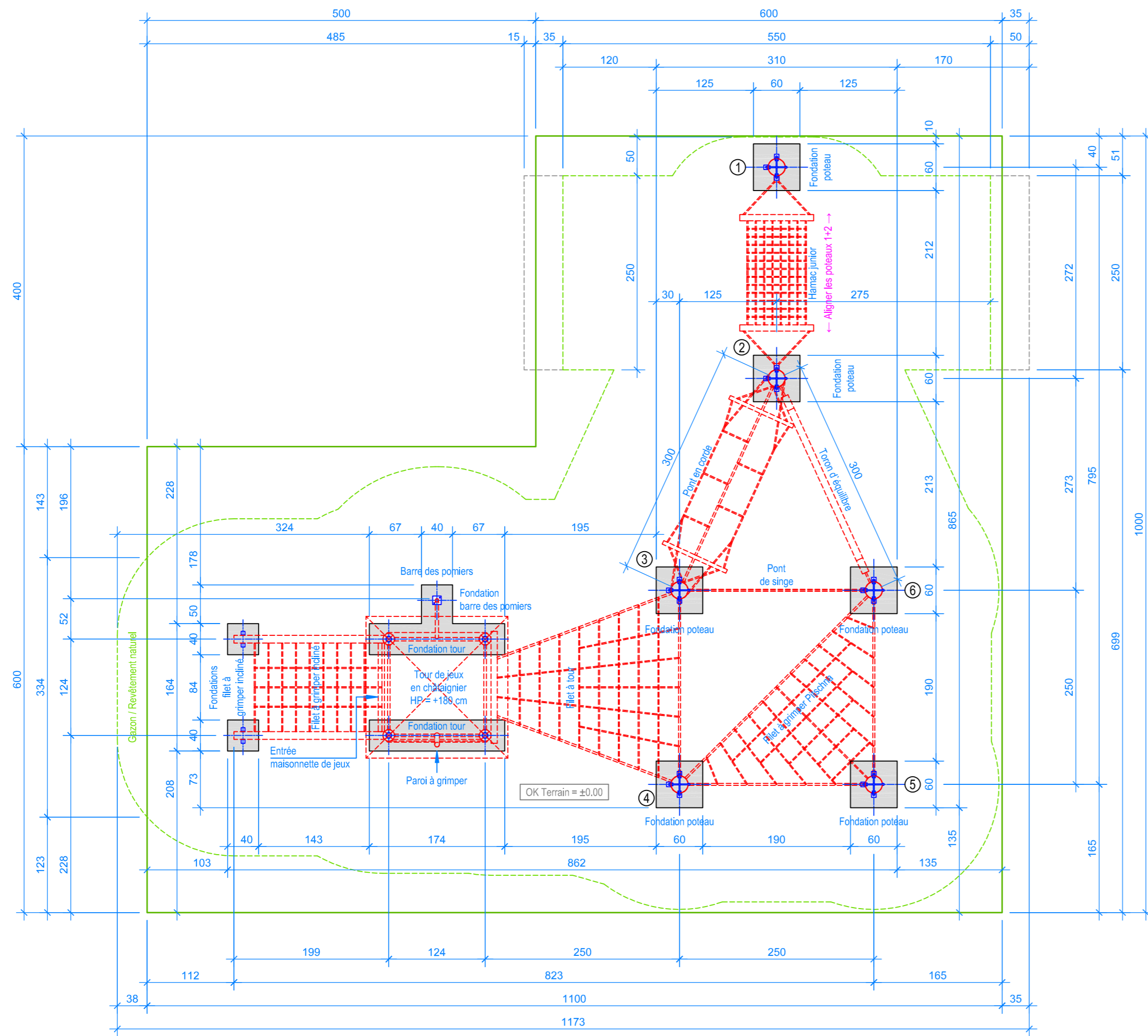
PLAN 1:50
