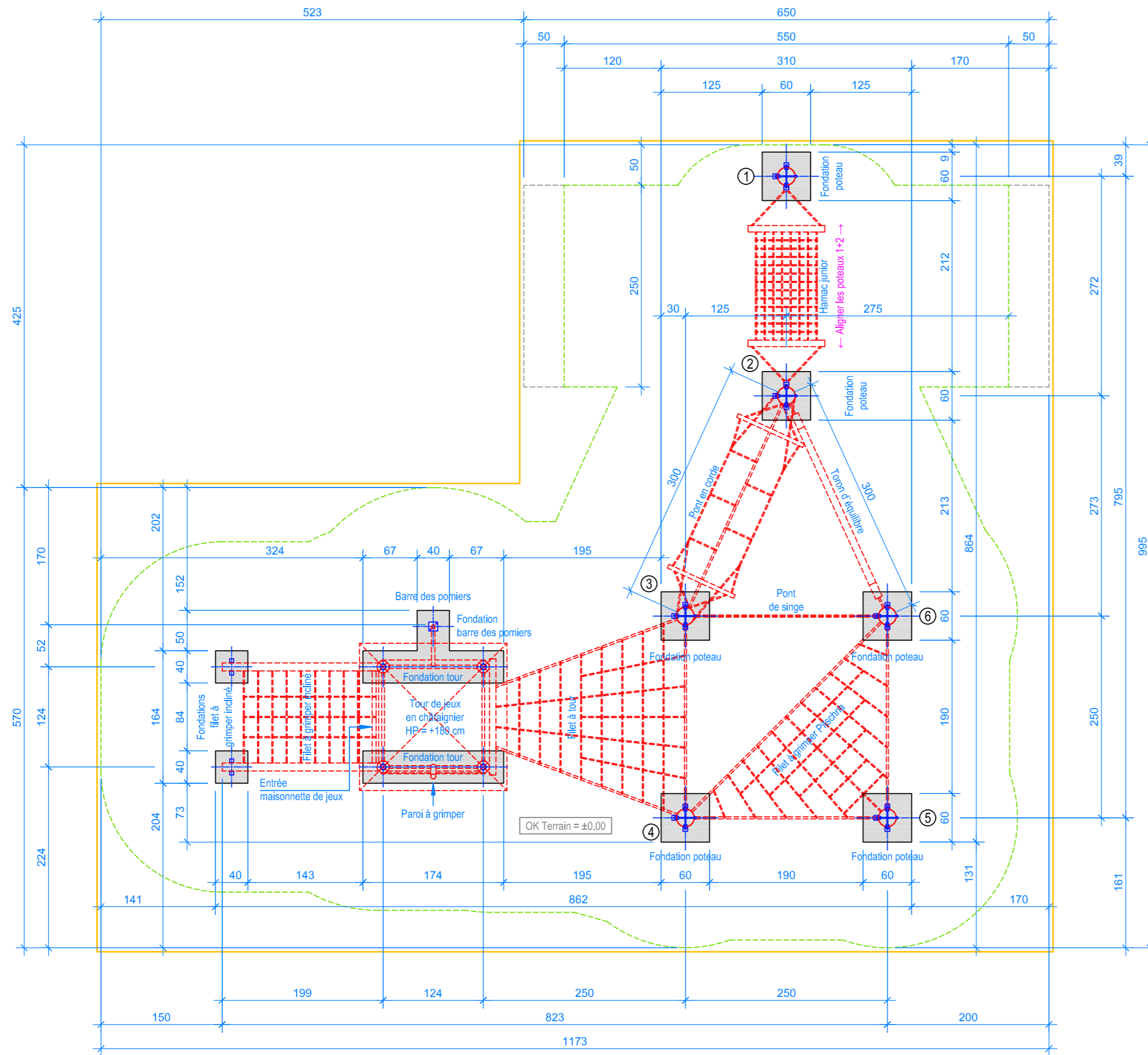
PLAN 1:50
