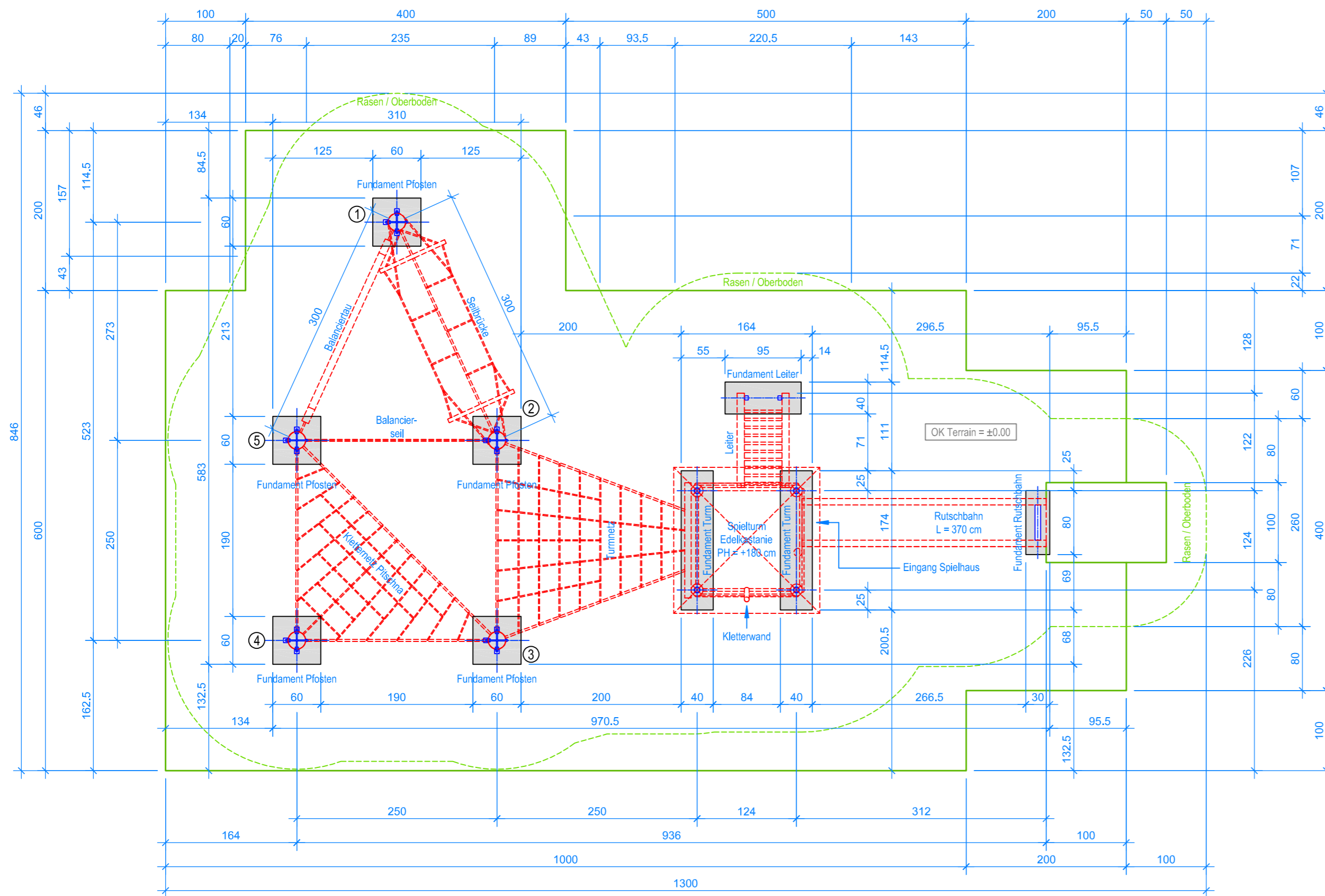
GRUNDRISS 1:50
