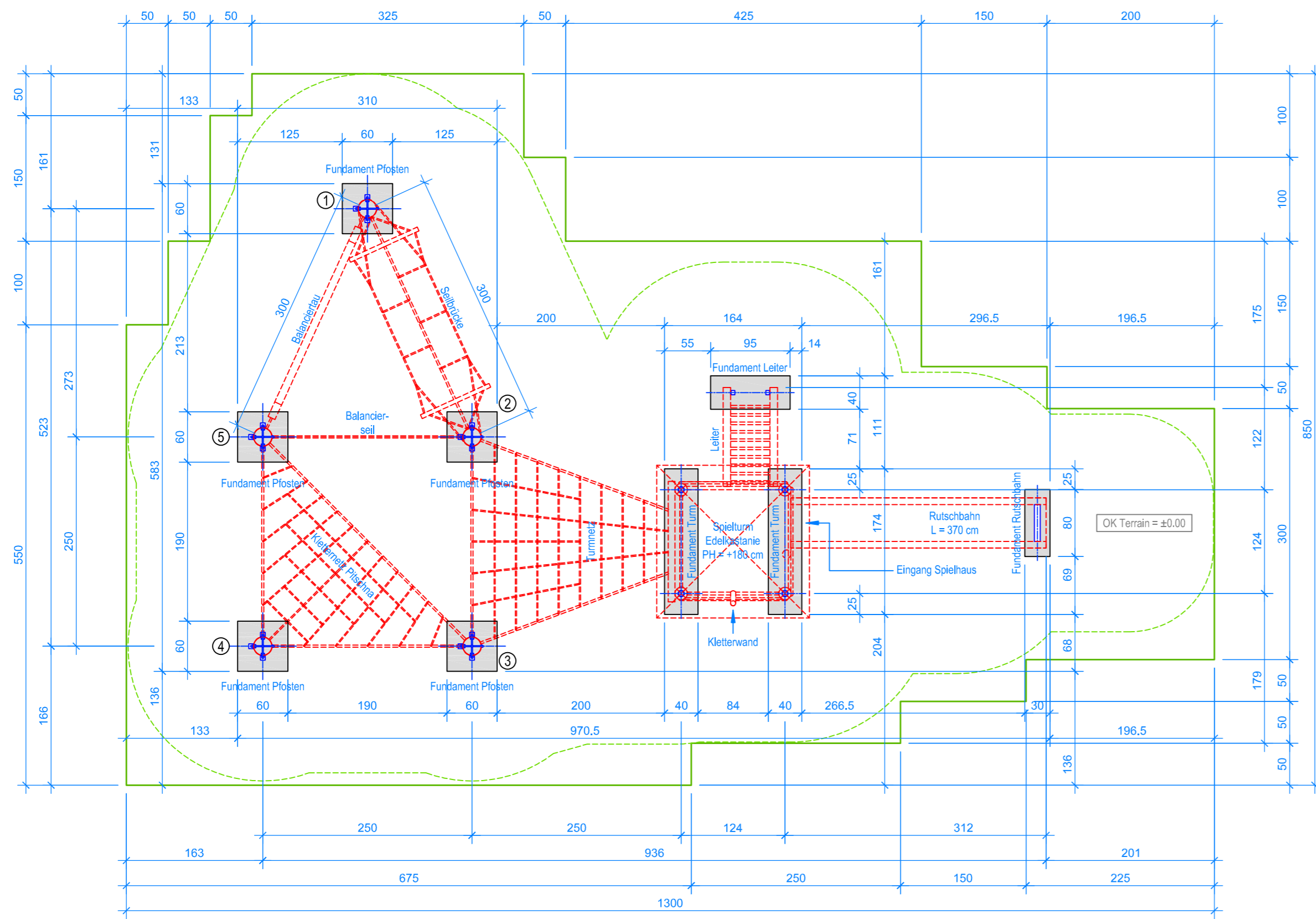
GRUNDRISS 1:50
