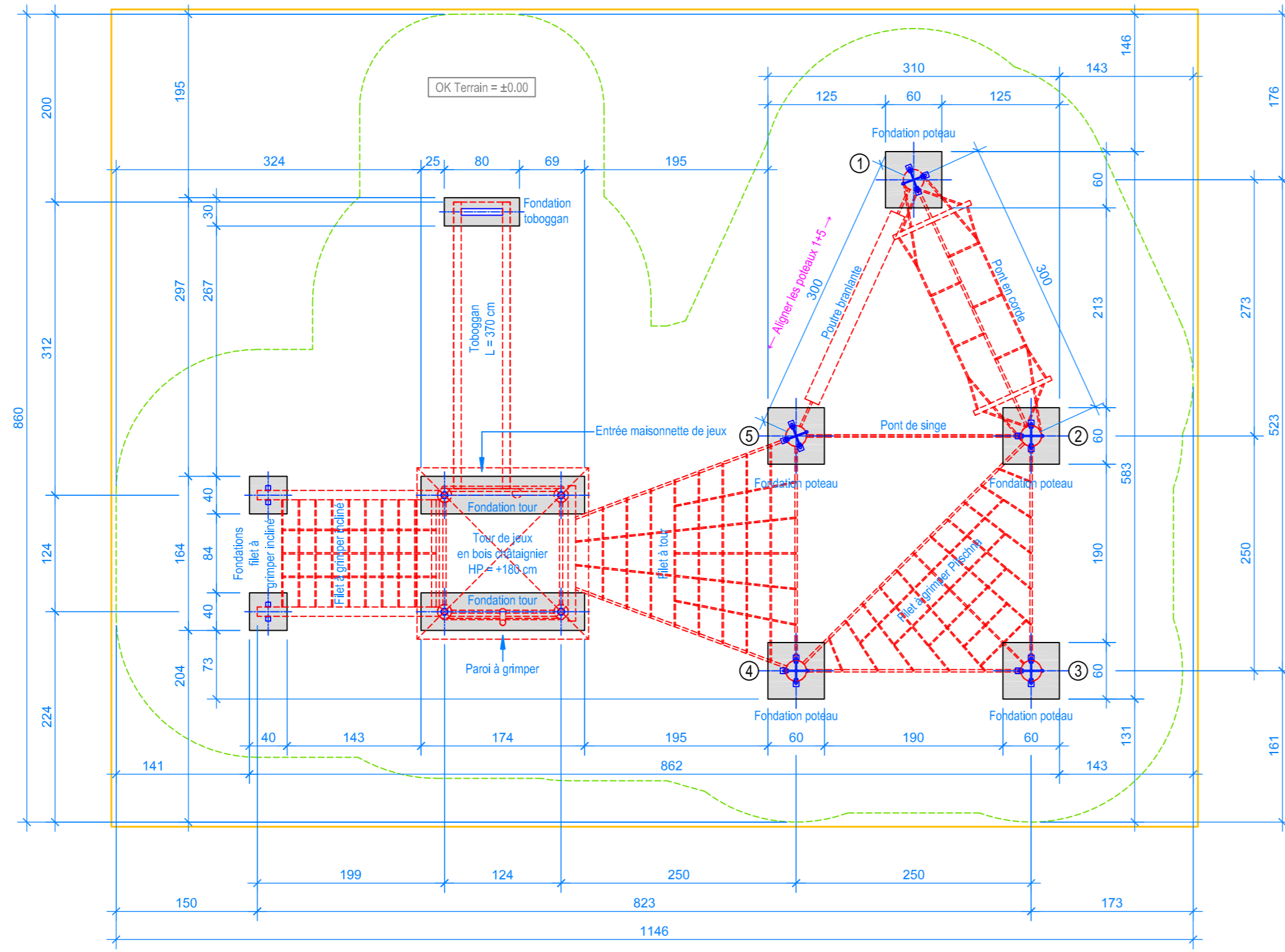
PLAN 1:50
