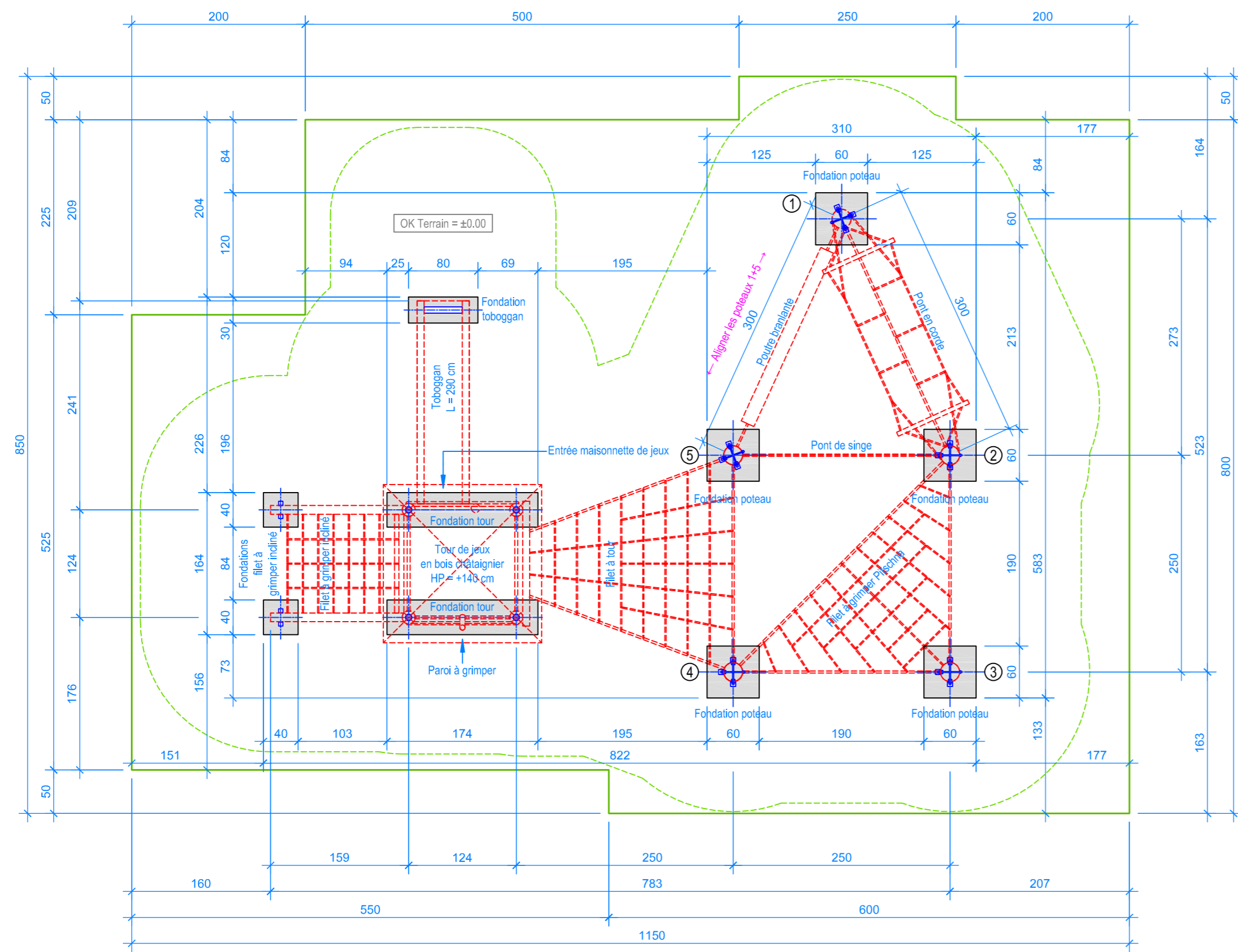
PLAN 1:50
