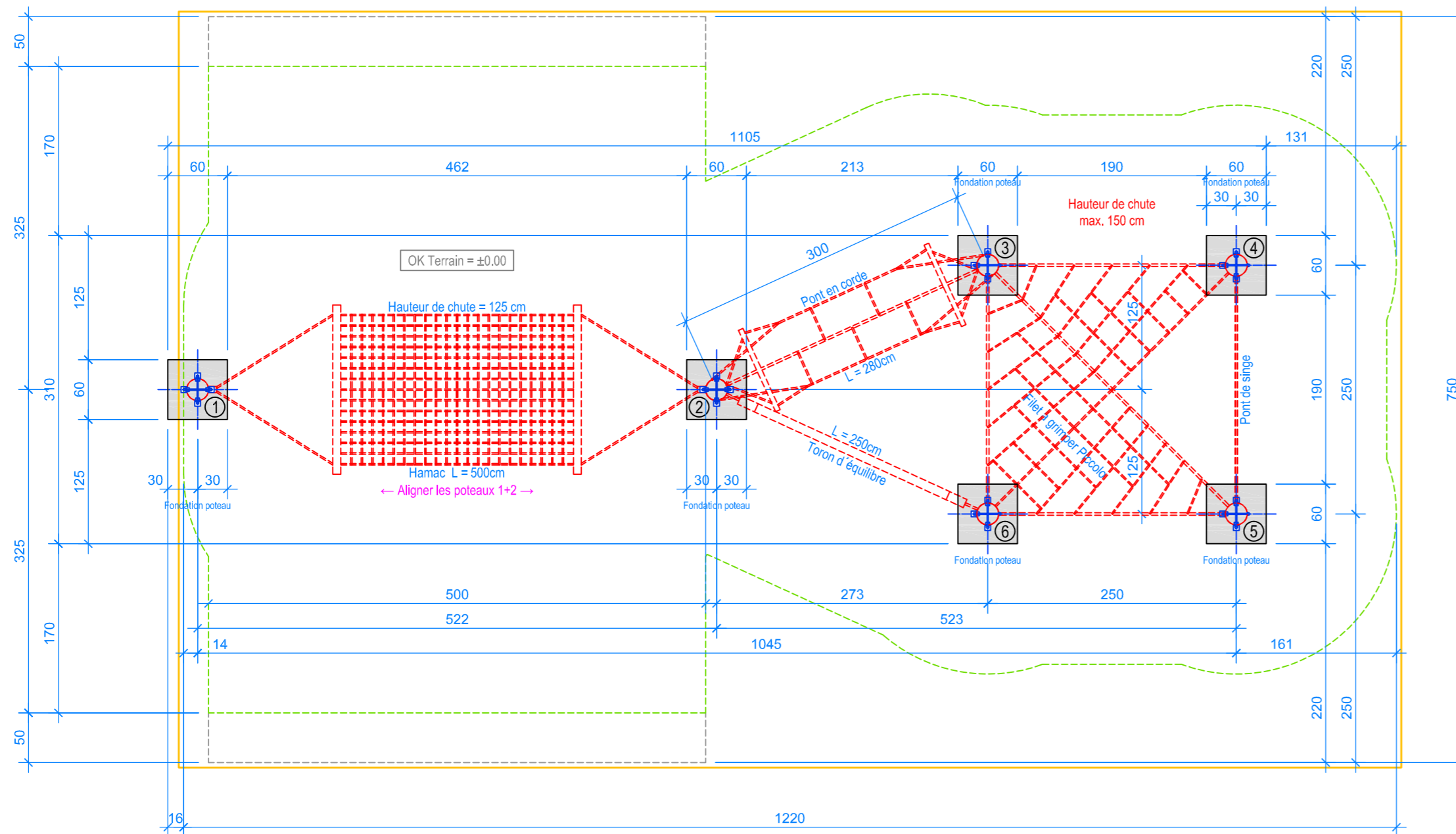
PLAN 1:50
