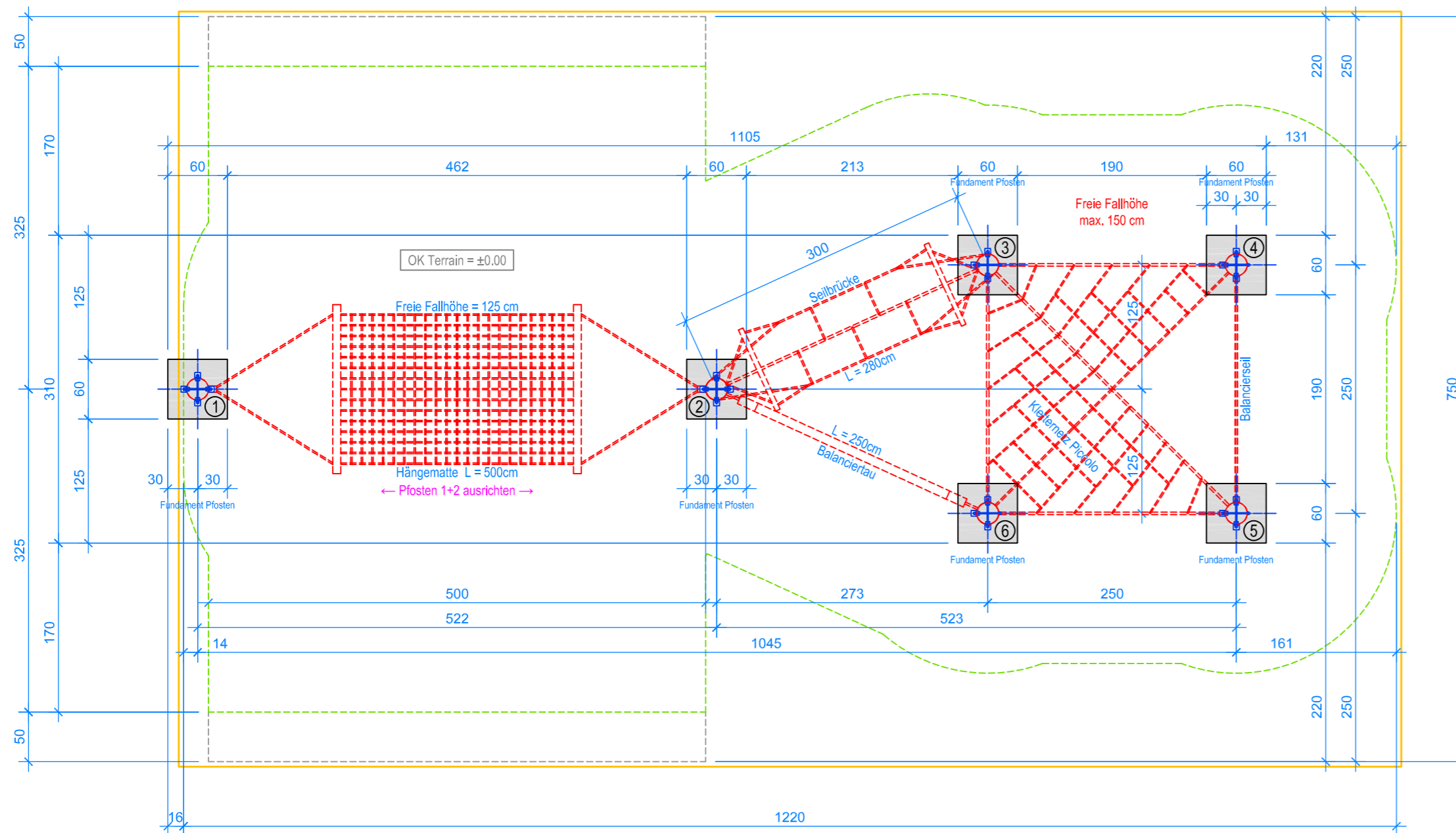
GRUNDRISS 1:50
