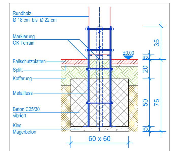
SCHNITT 1:20 FUNDAMENT PFOSTEN 1-6
