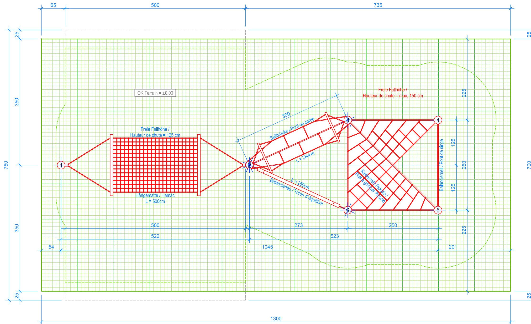
GRUNDRISS / PLAN 1:50
