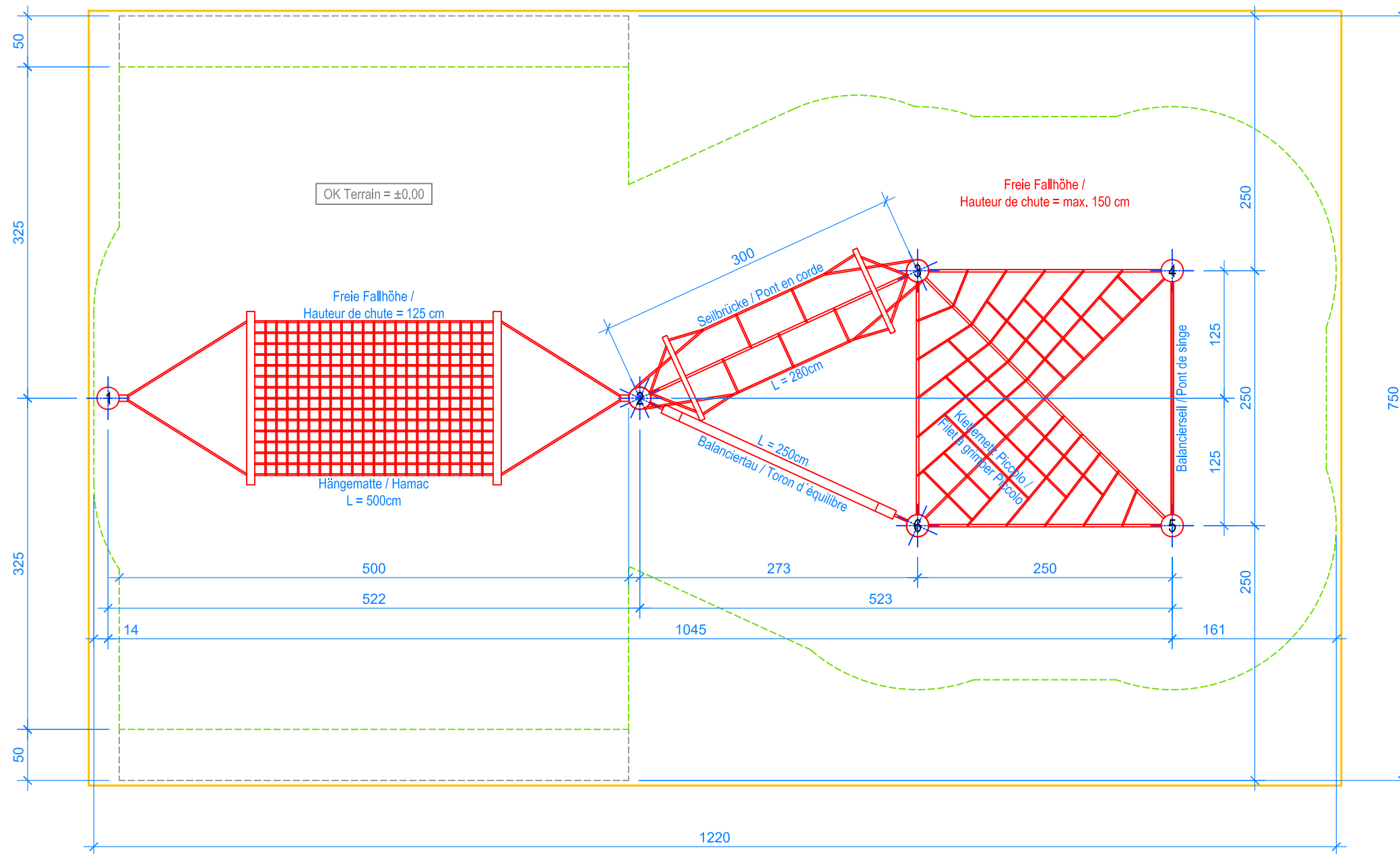
GRUNDRISS / PLAN 1:50
