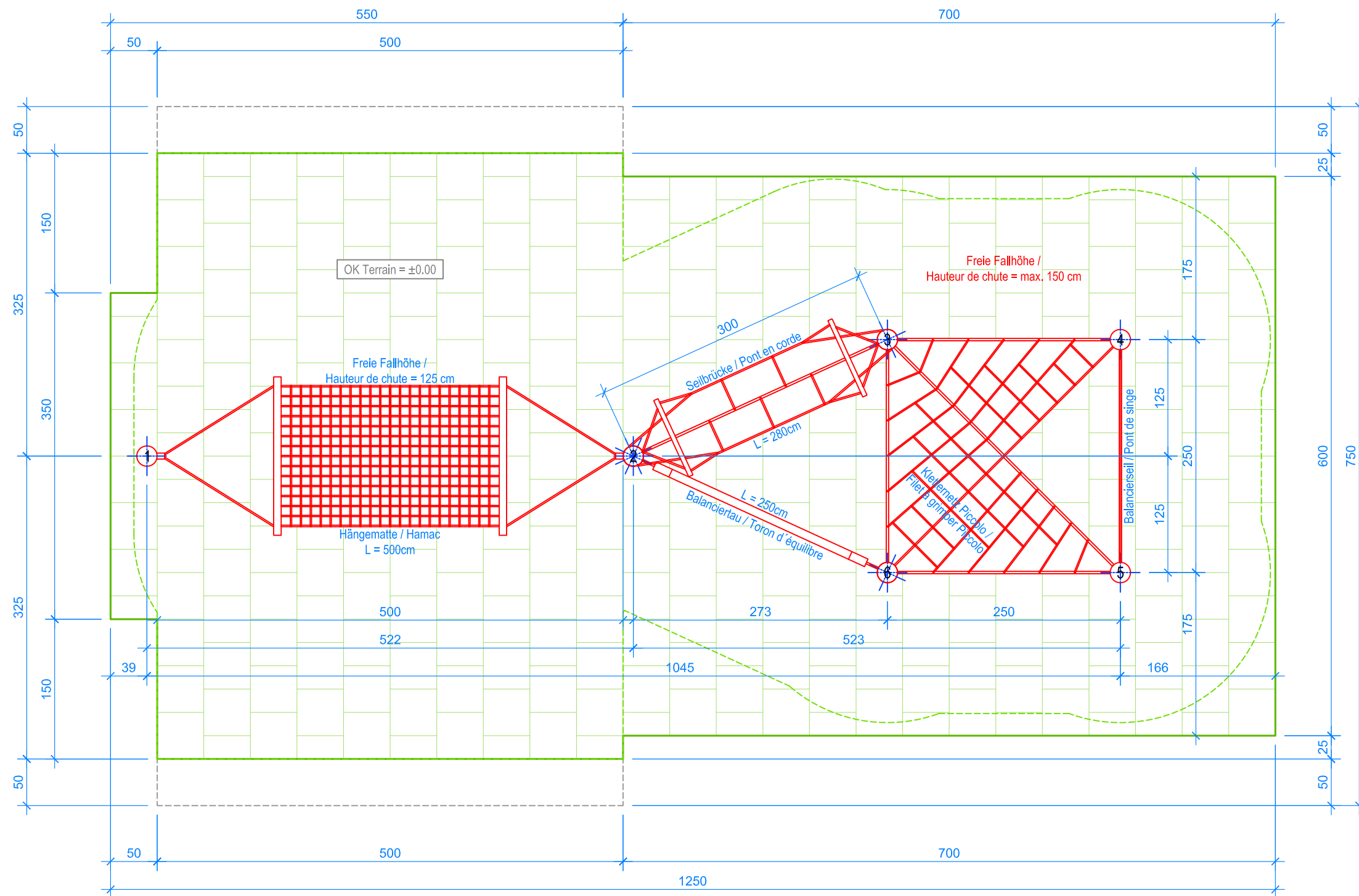
GRUNDRISS / PLAN 1:50
