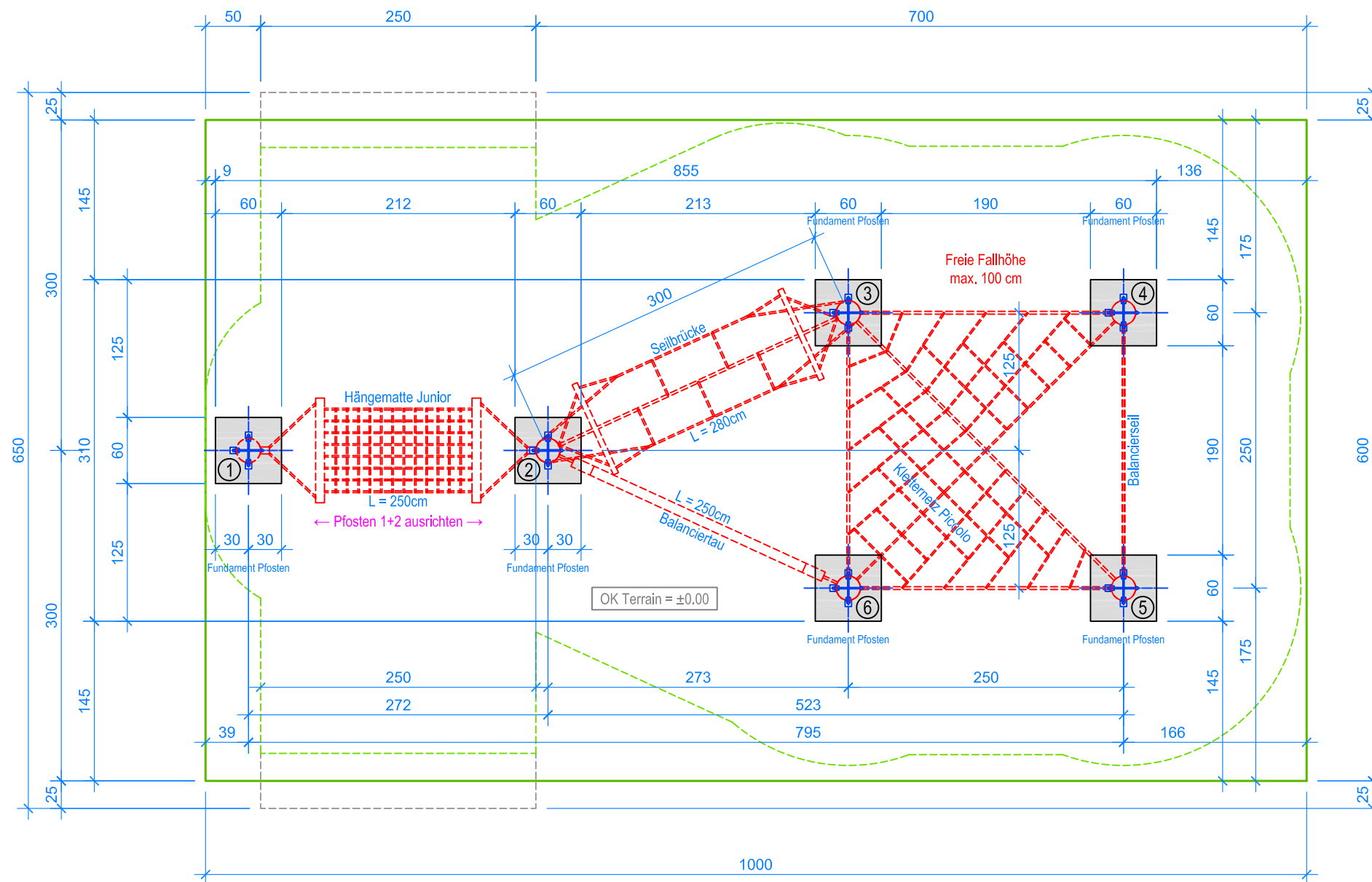
GRUNDRISS 1:50
