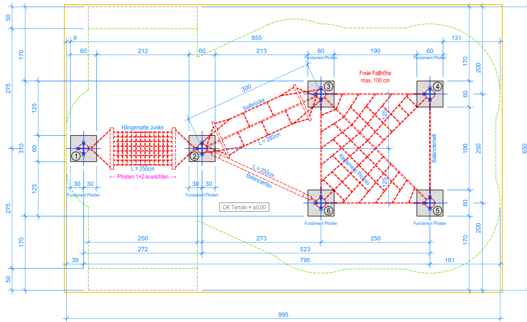
GRUNDRISS 1:50
