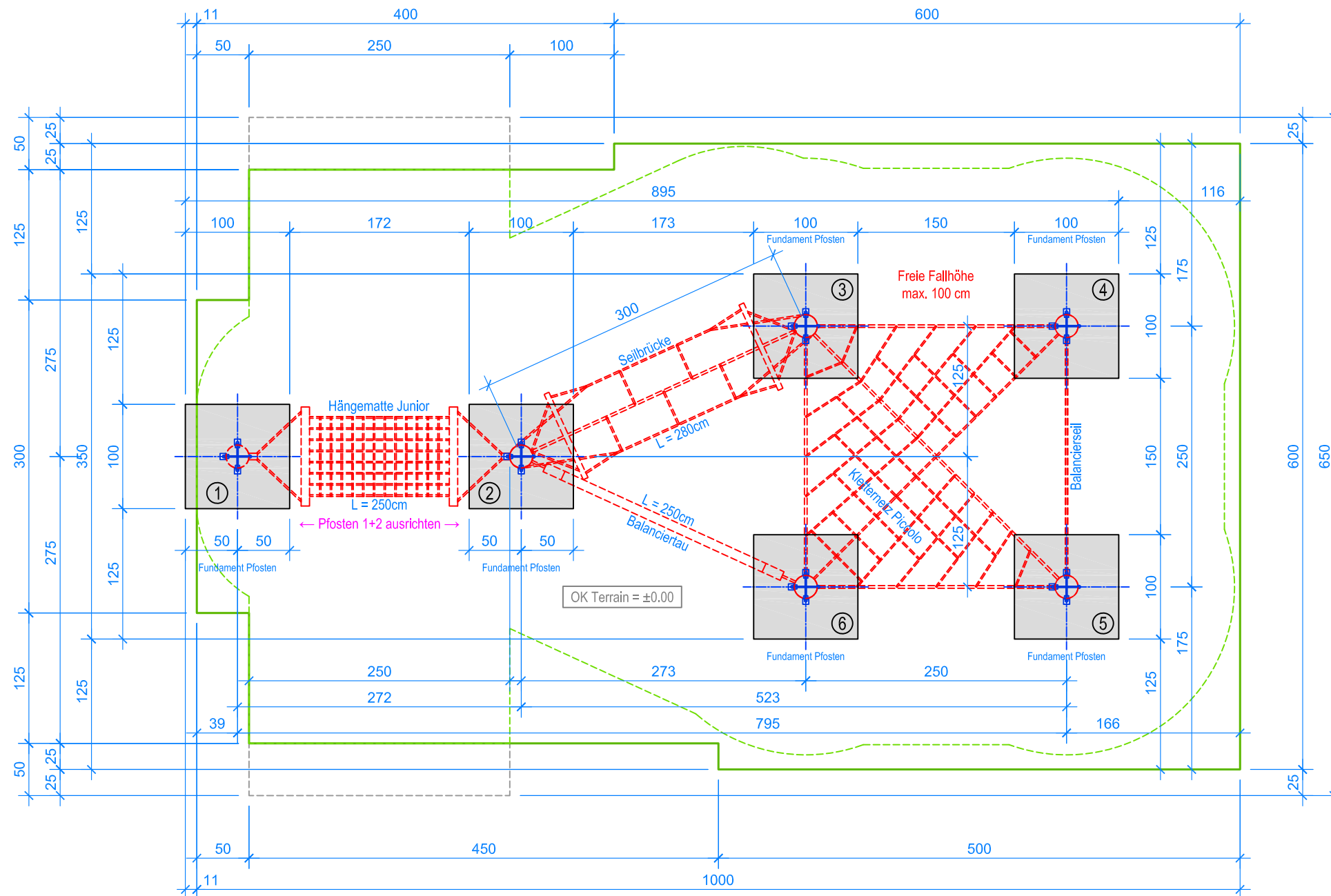
GRUNDRISS 1:50
