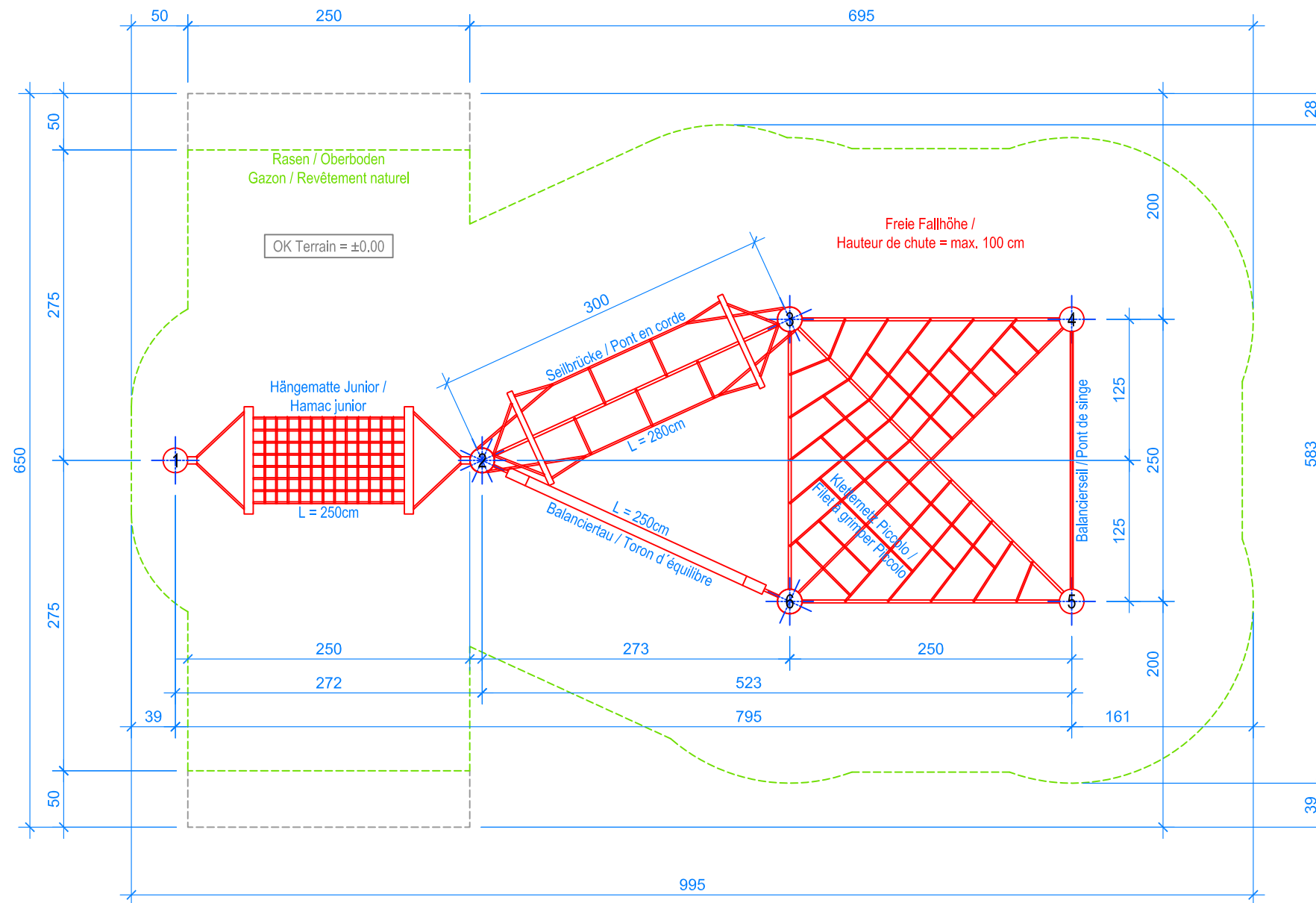
GRUNDRISS / PLAN 1:50
