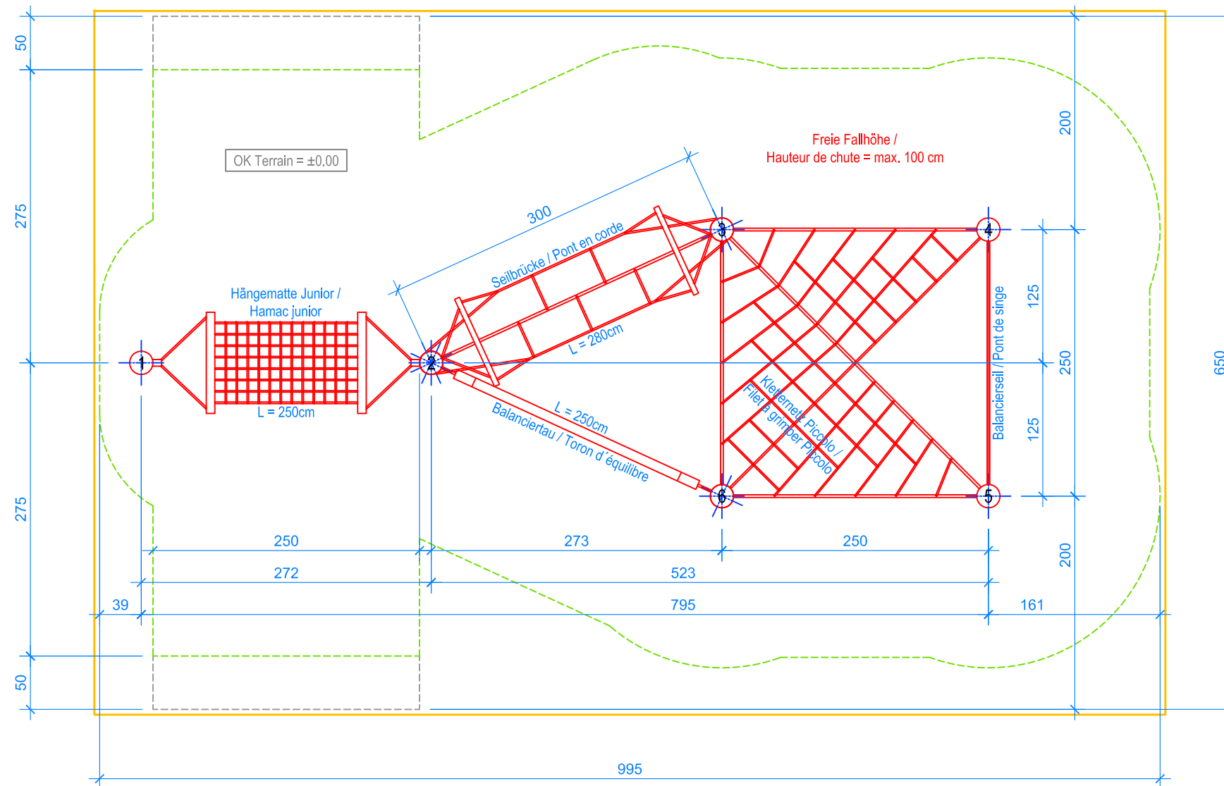
GRUNDRISS / PLAN 1:50
