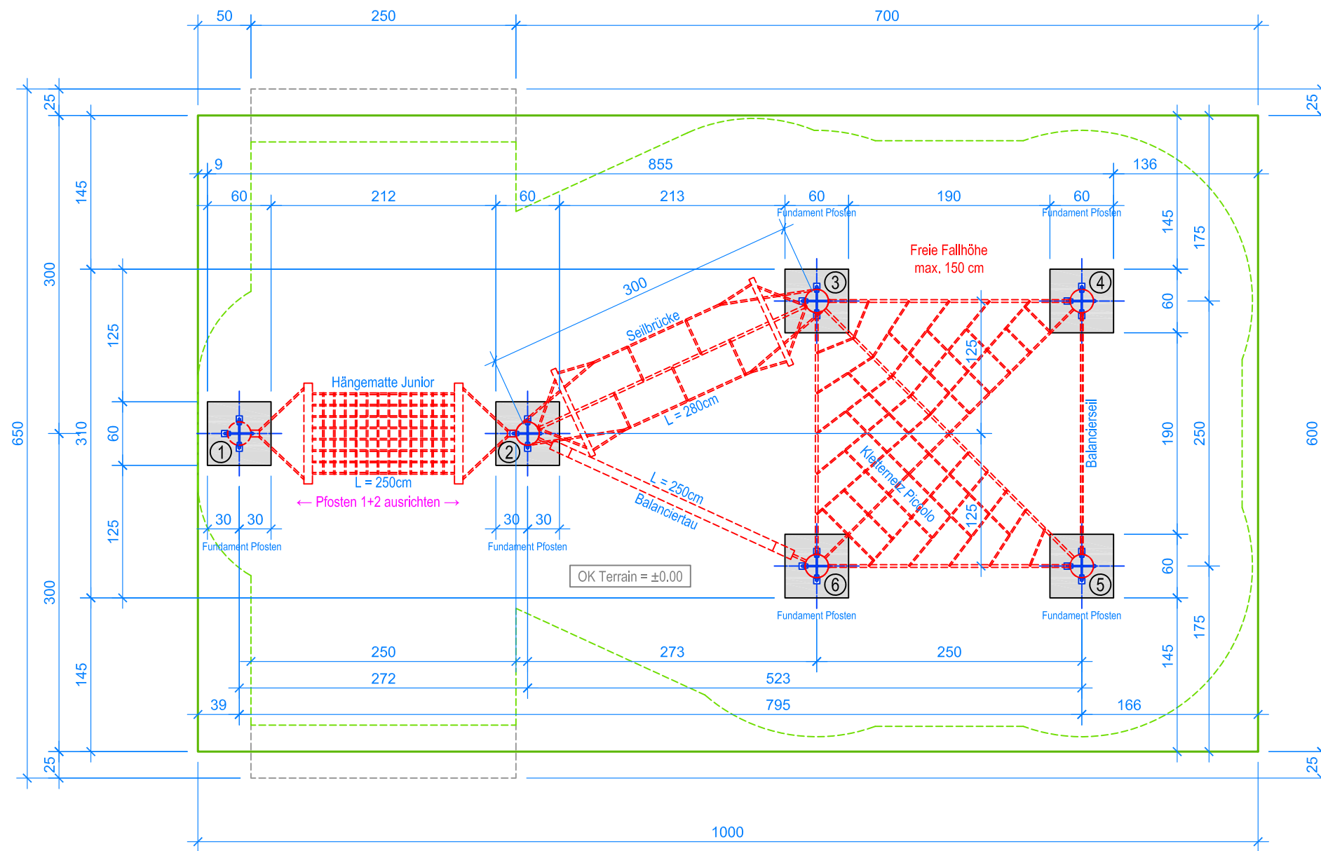
GRUNDRISS 1:50
