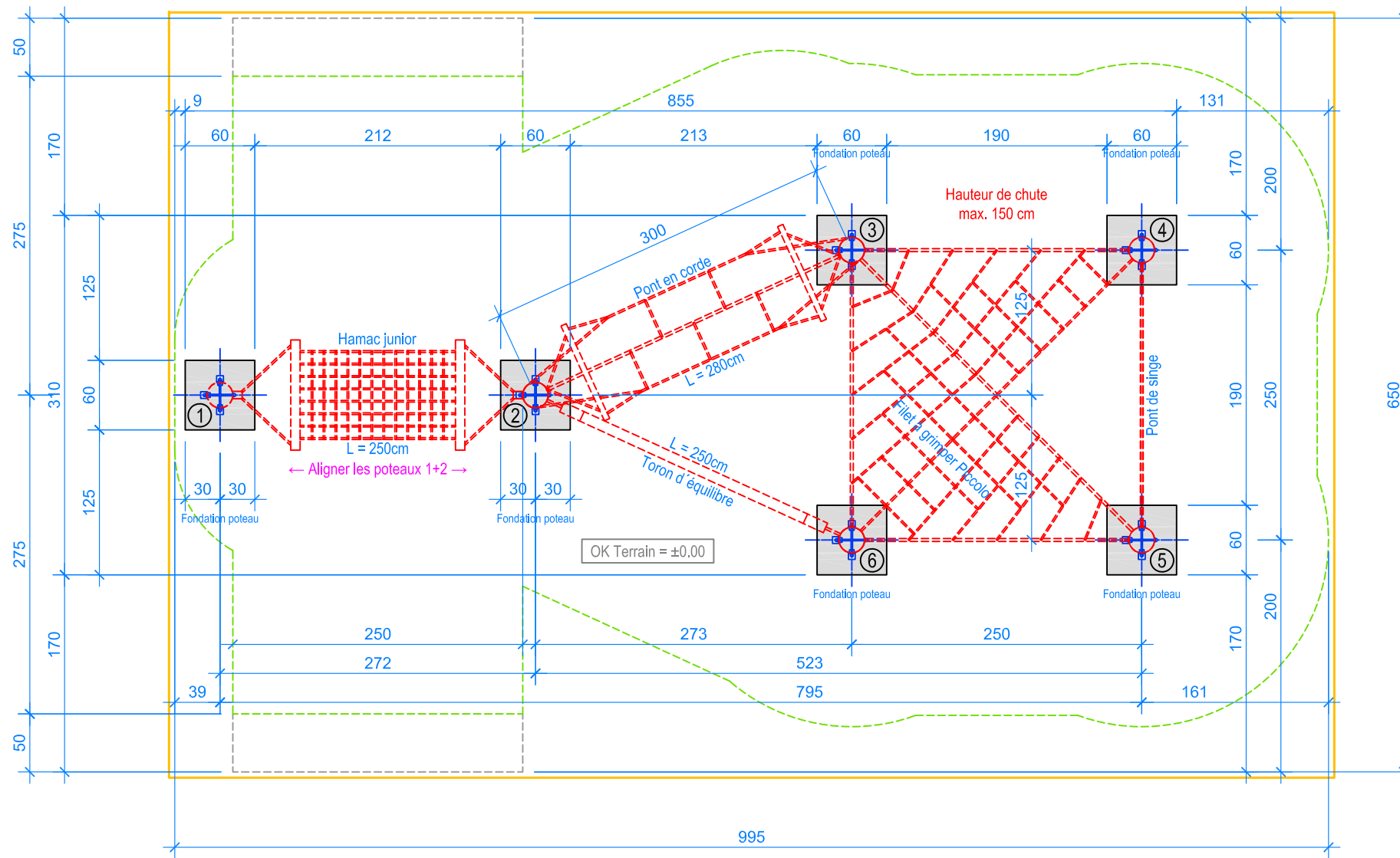
PLAN 1:50
