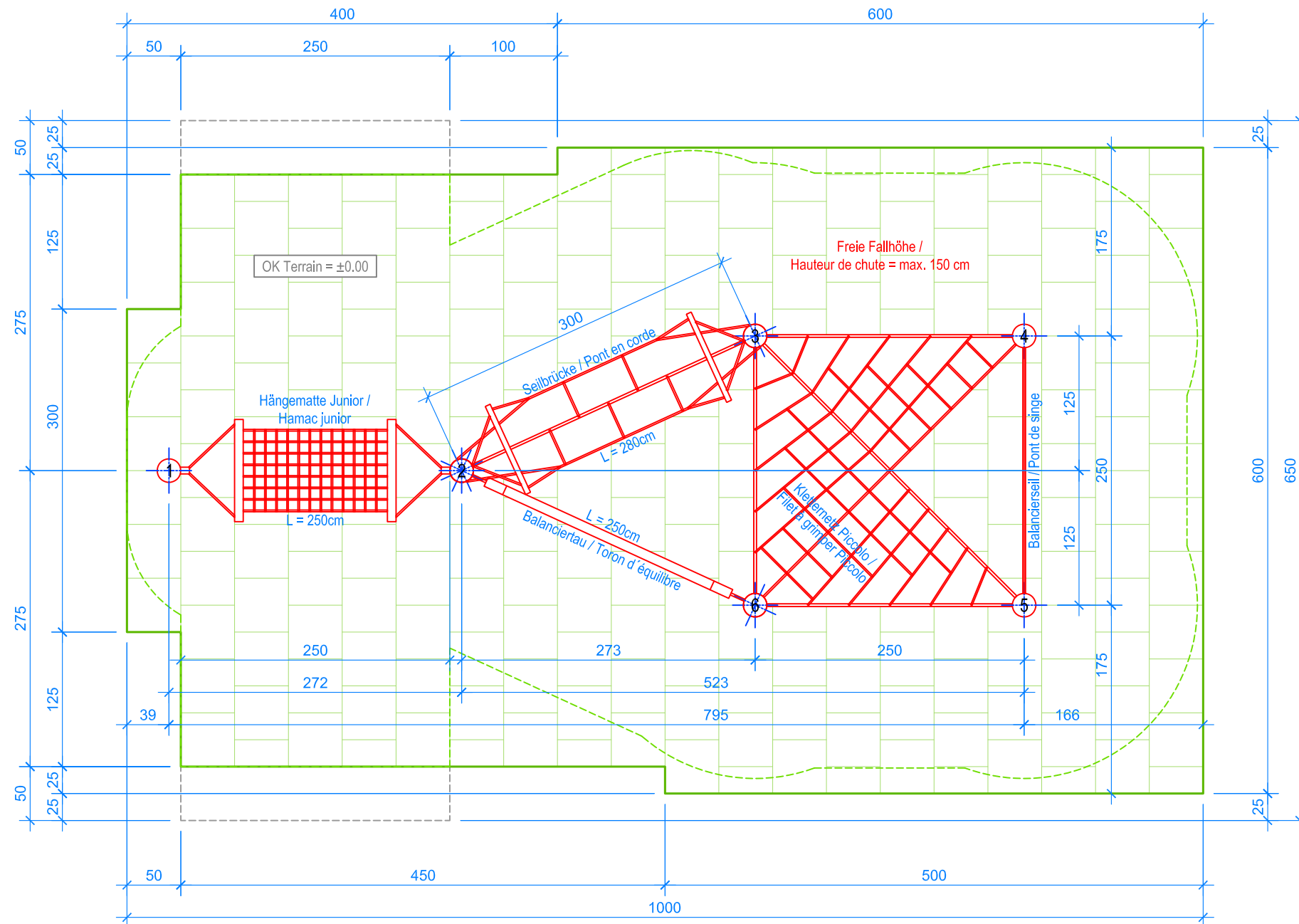
GRUNDRISS / PLAN 1:50
