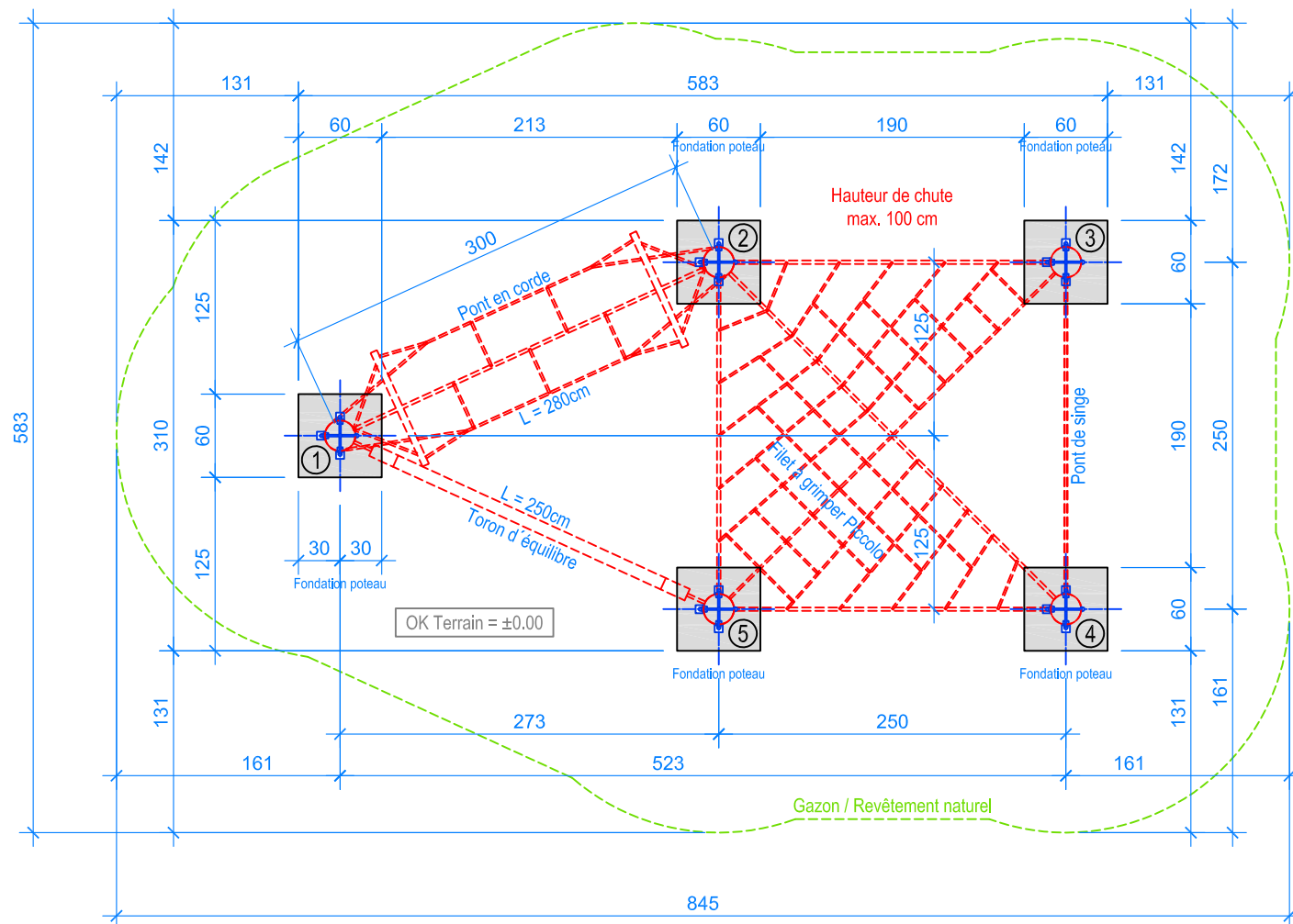
PLAN 1:50
