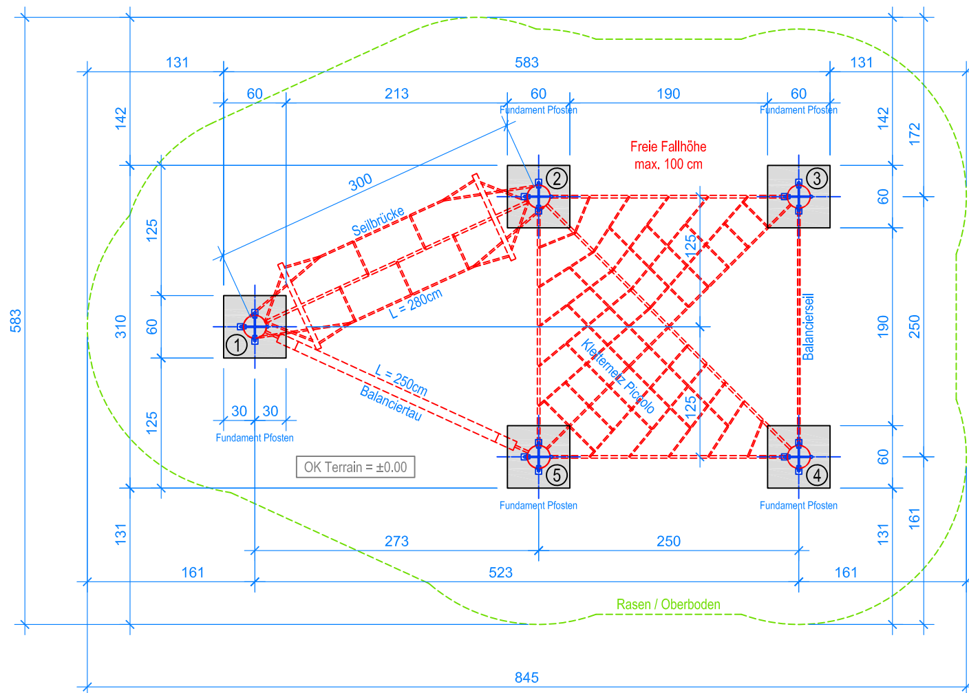
GRUNDRISS 1:50
