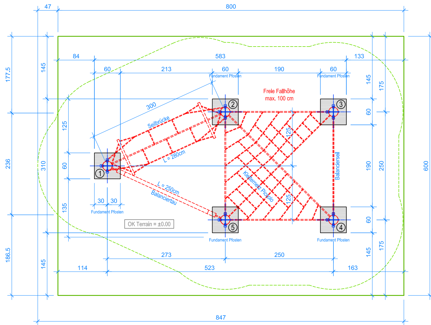
GRUNDRISS 1:50
