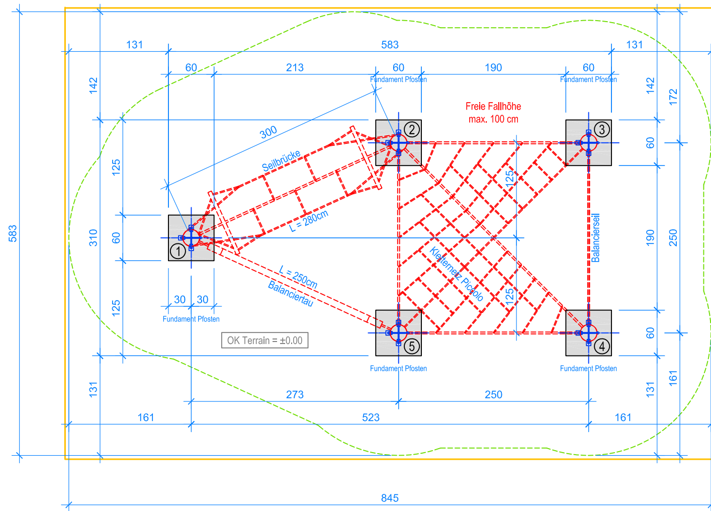
GRUNDRISS 1:50
