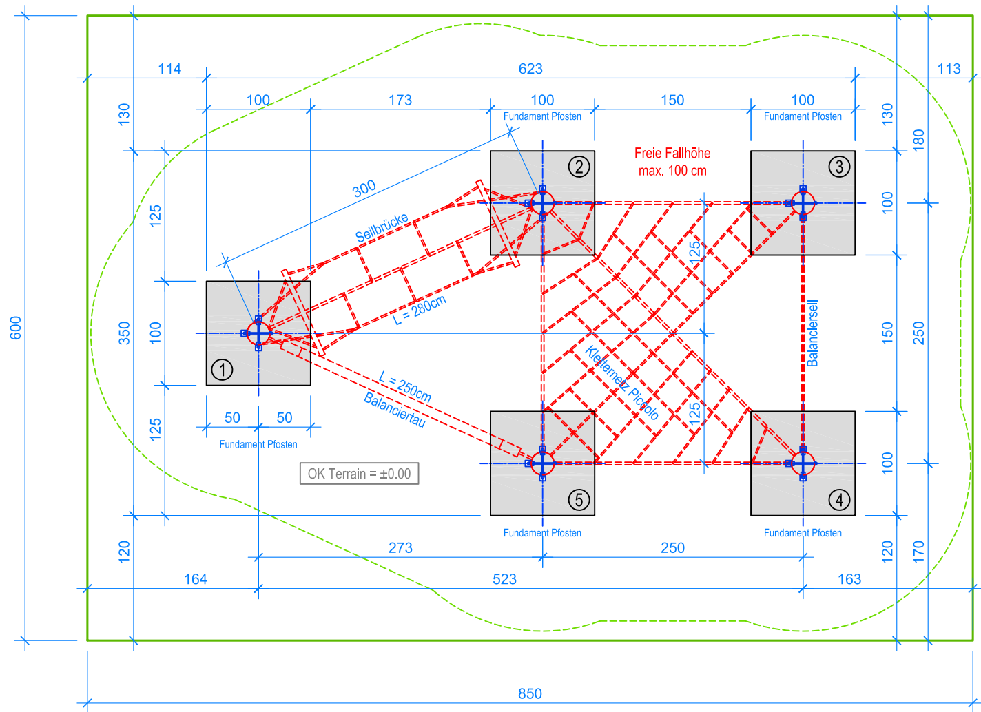
GRUNDRISS 1:50
