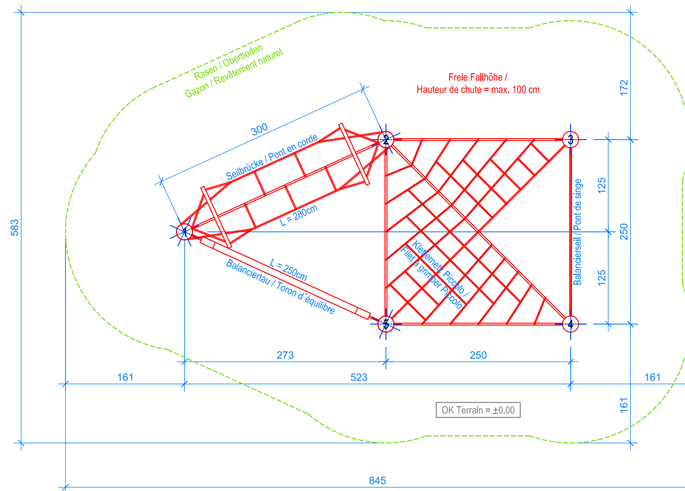
GRUNDRISS / PLAN 1:50
