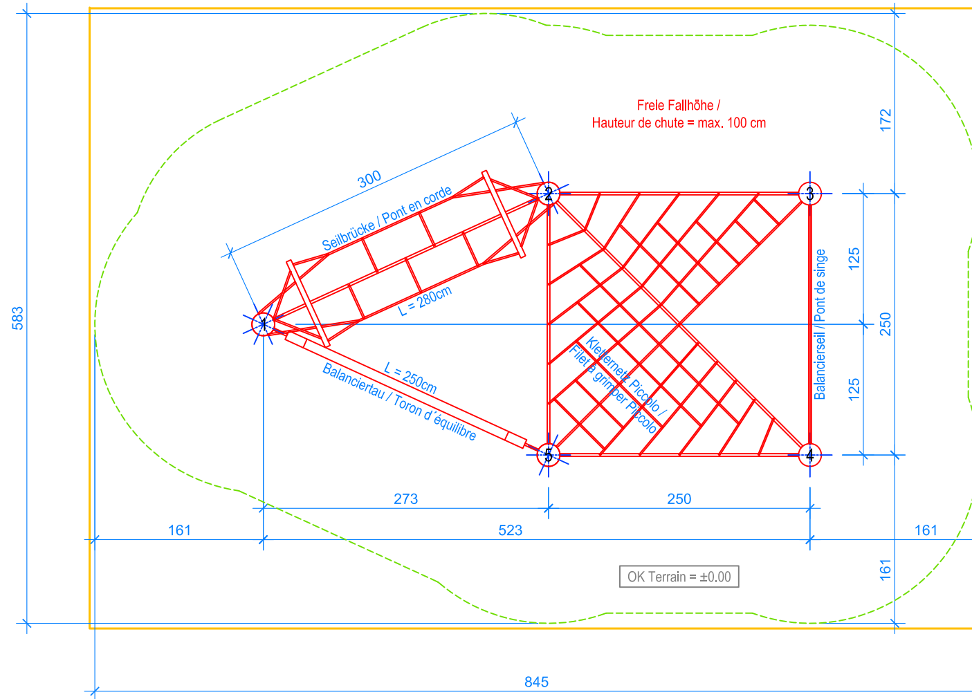
GRUNDRISS / PLAN 1:50
