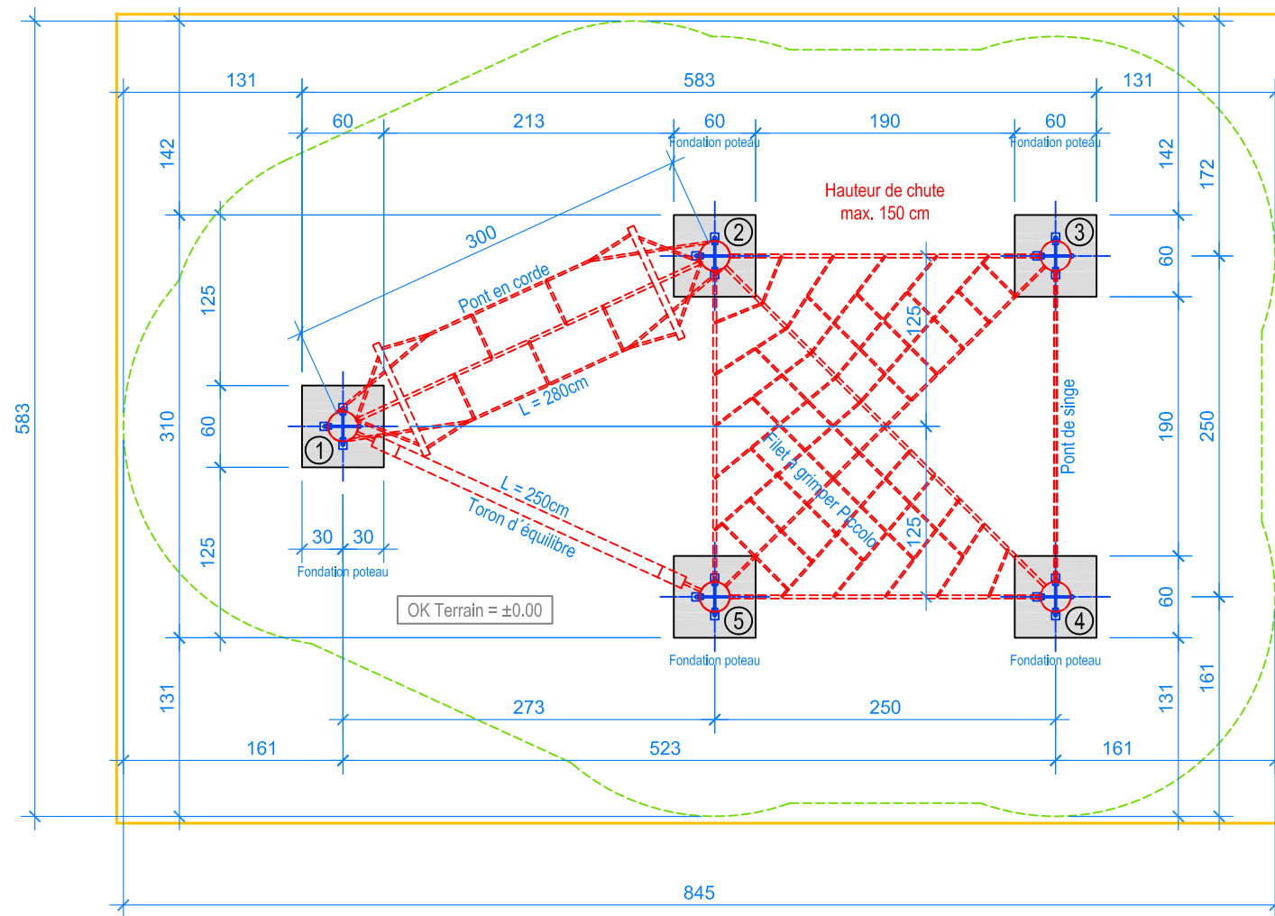
PLAN 1:50
