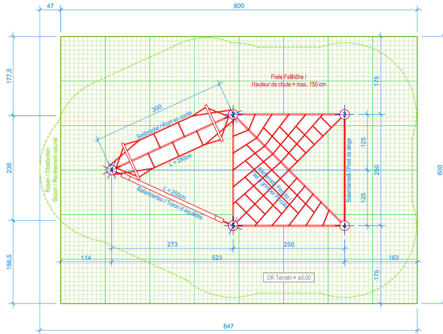
GRUNDRISS / PLAN 1:50
