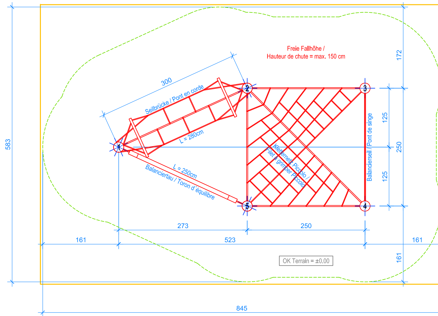
GRUNDRISS / PLAN 1:50
