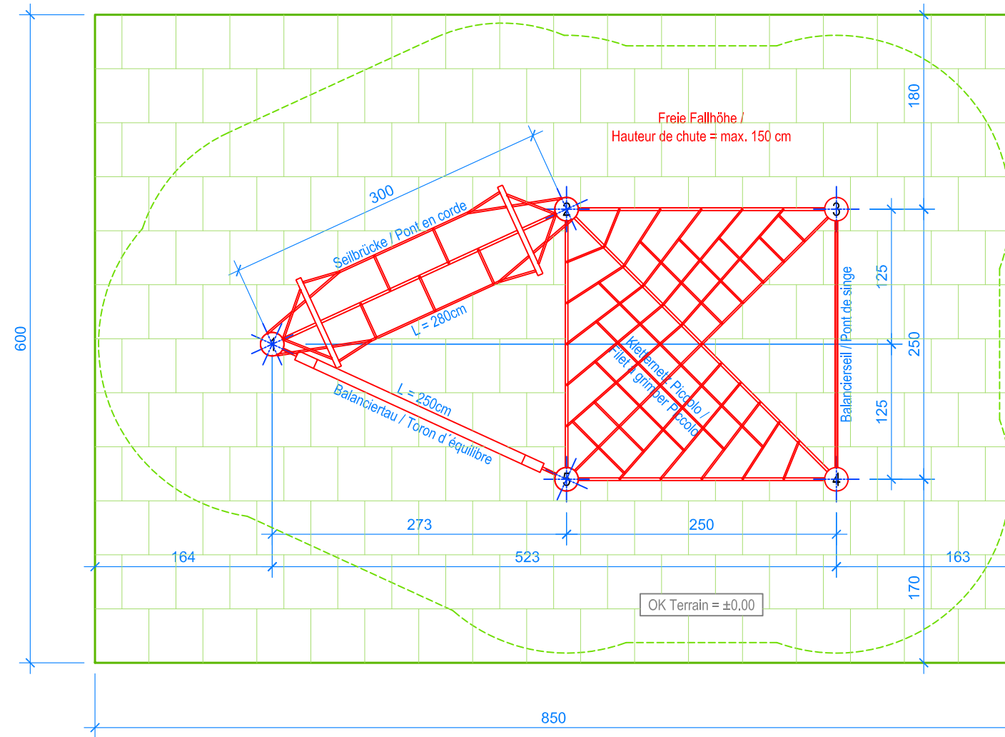
GRUNDRISS / PLAN 1:50
