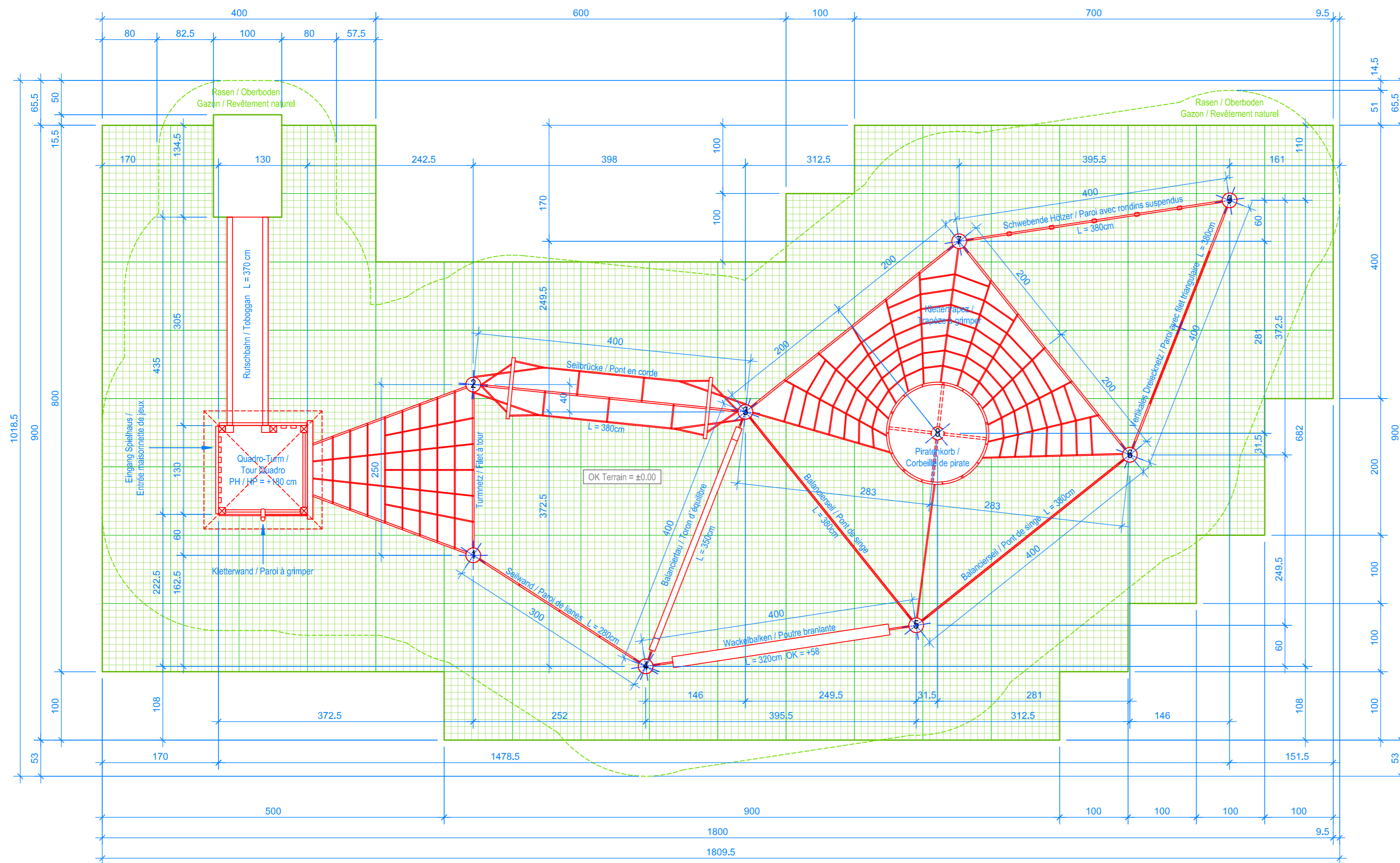
GRUNDRISS / PLAN 1:50
