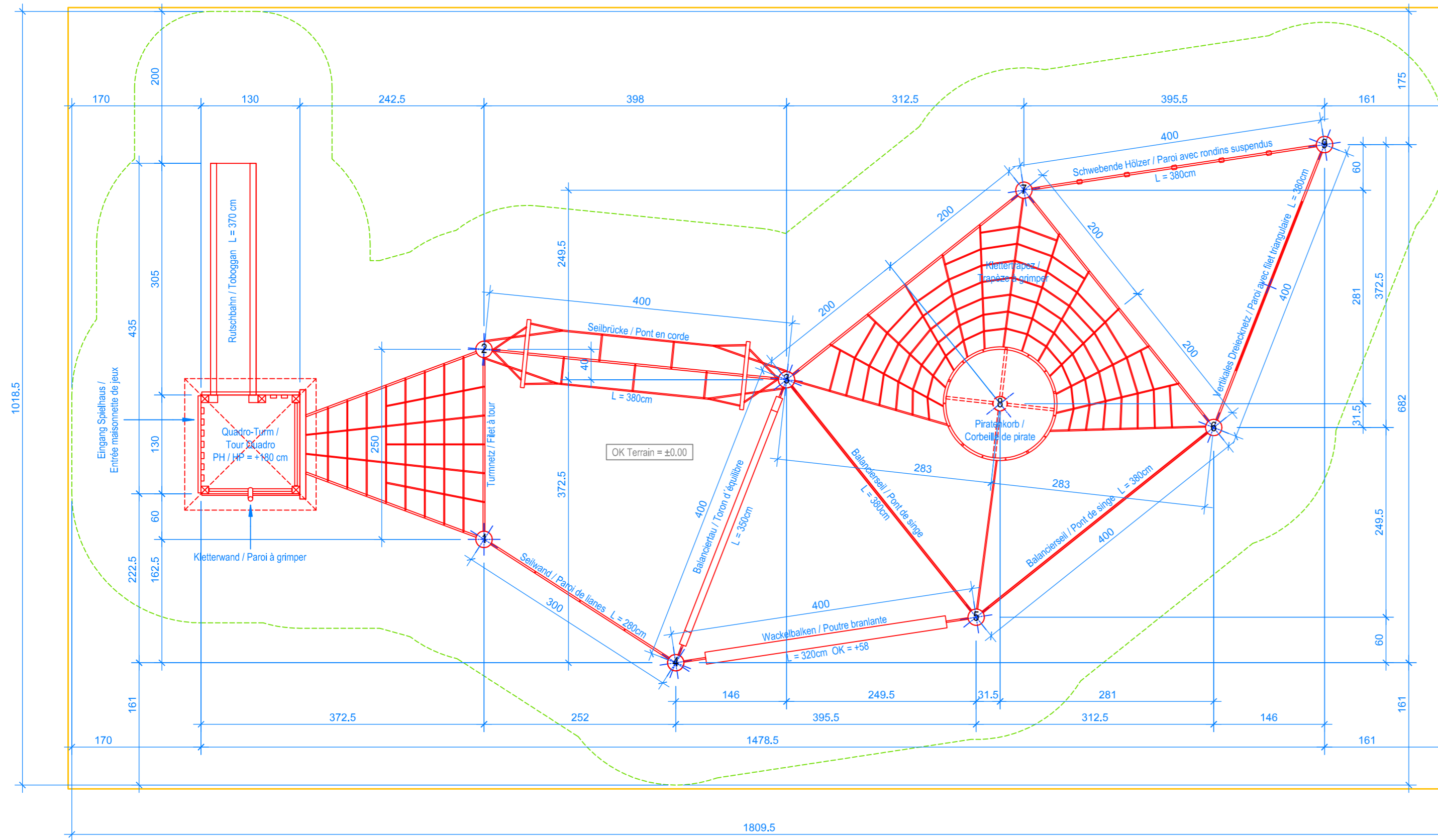
GRUNDRISS / PLAN 1:50
