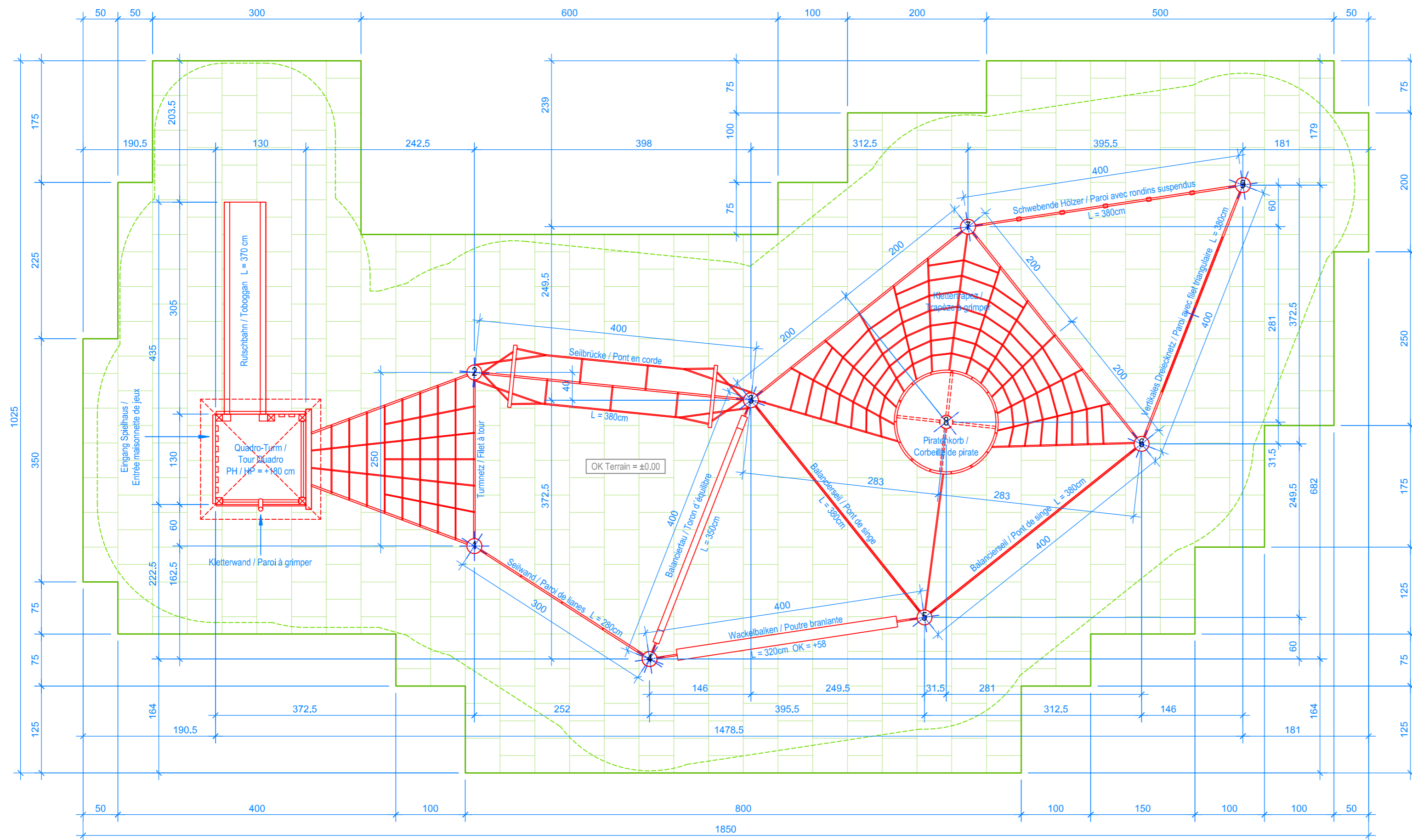
GRUNDRISS / PLAN 1:50
