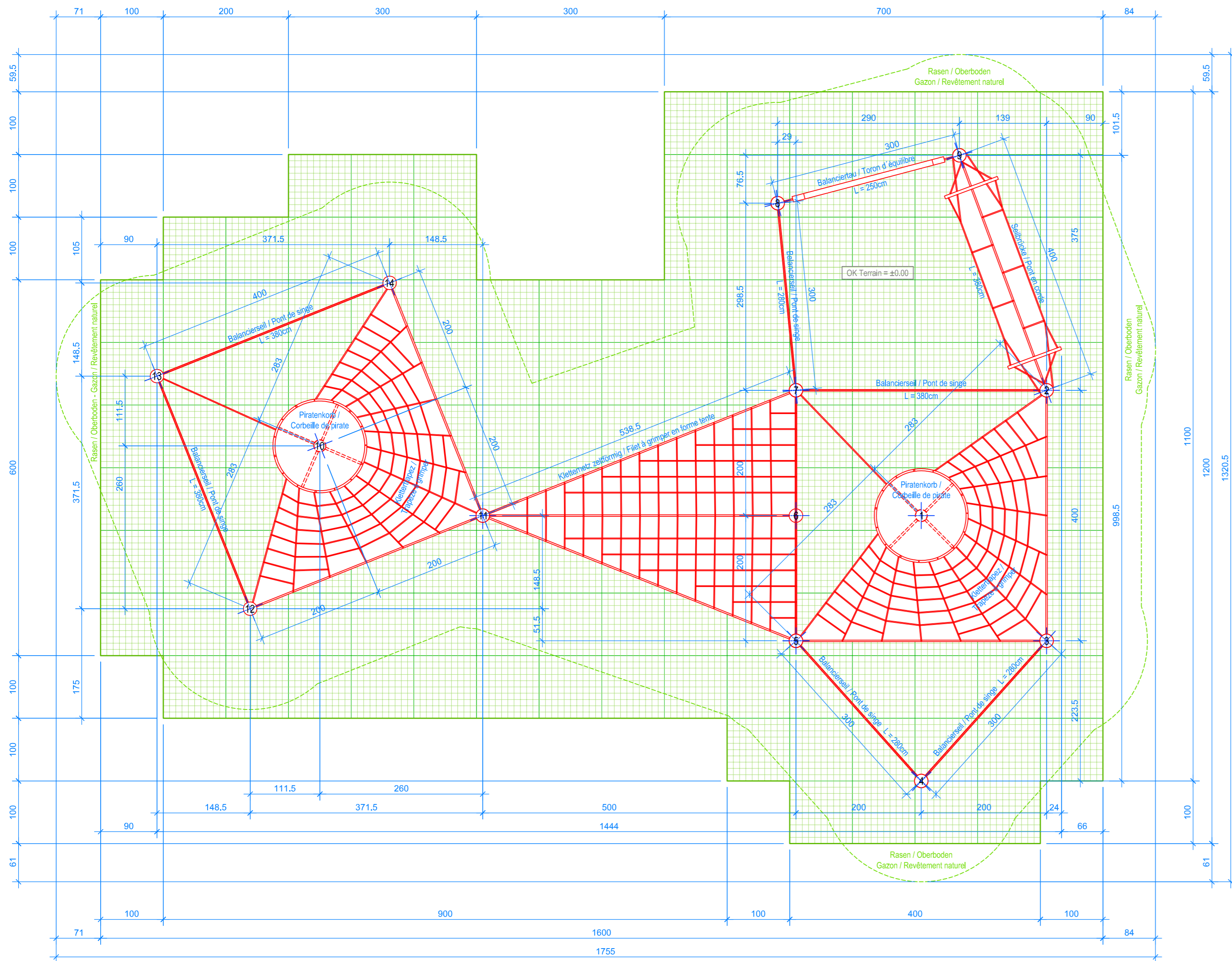
GRUNDRISS / PLAN 1:50
