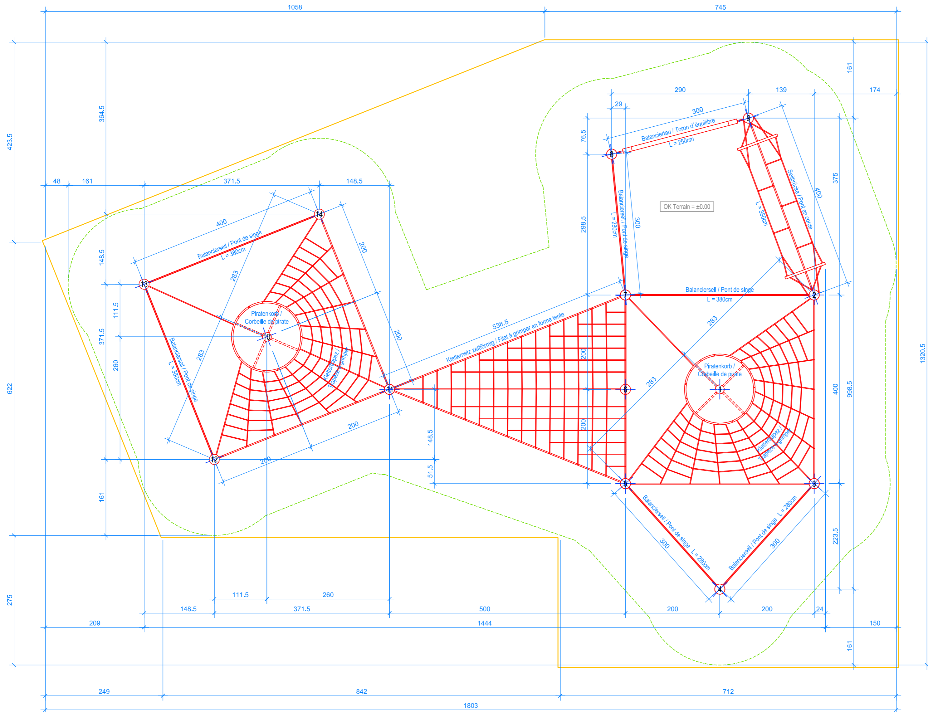
GRUNDRISS / PLAN 1:50
