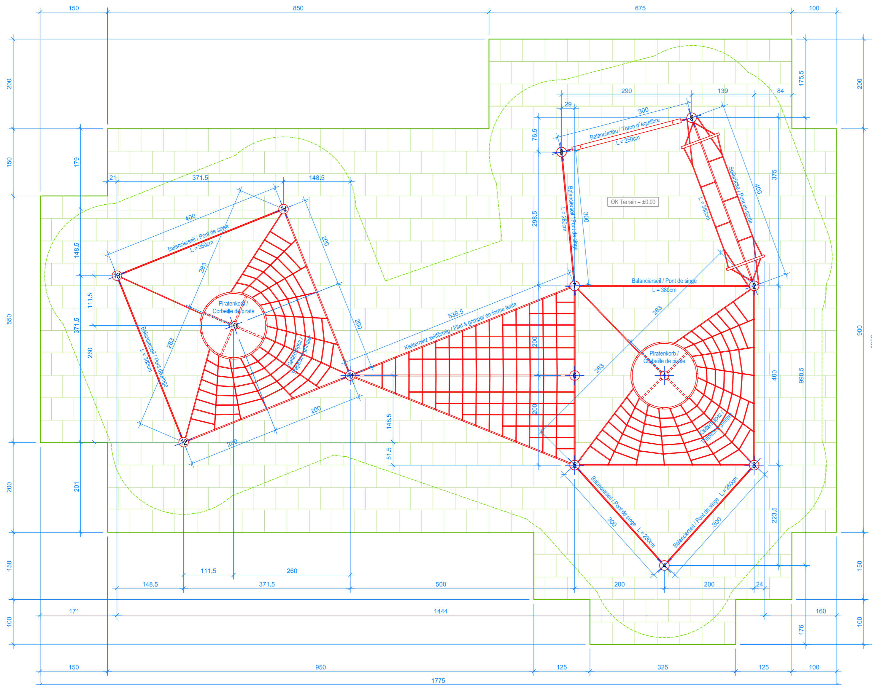
GRUNDRISS / PLAN 1:50
