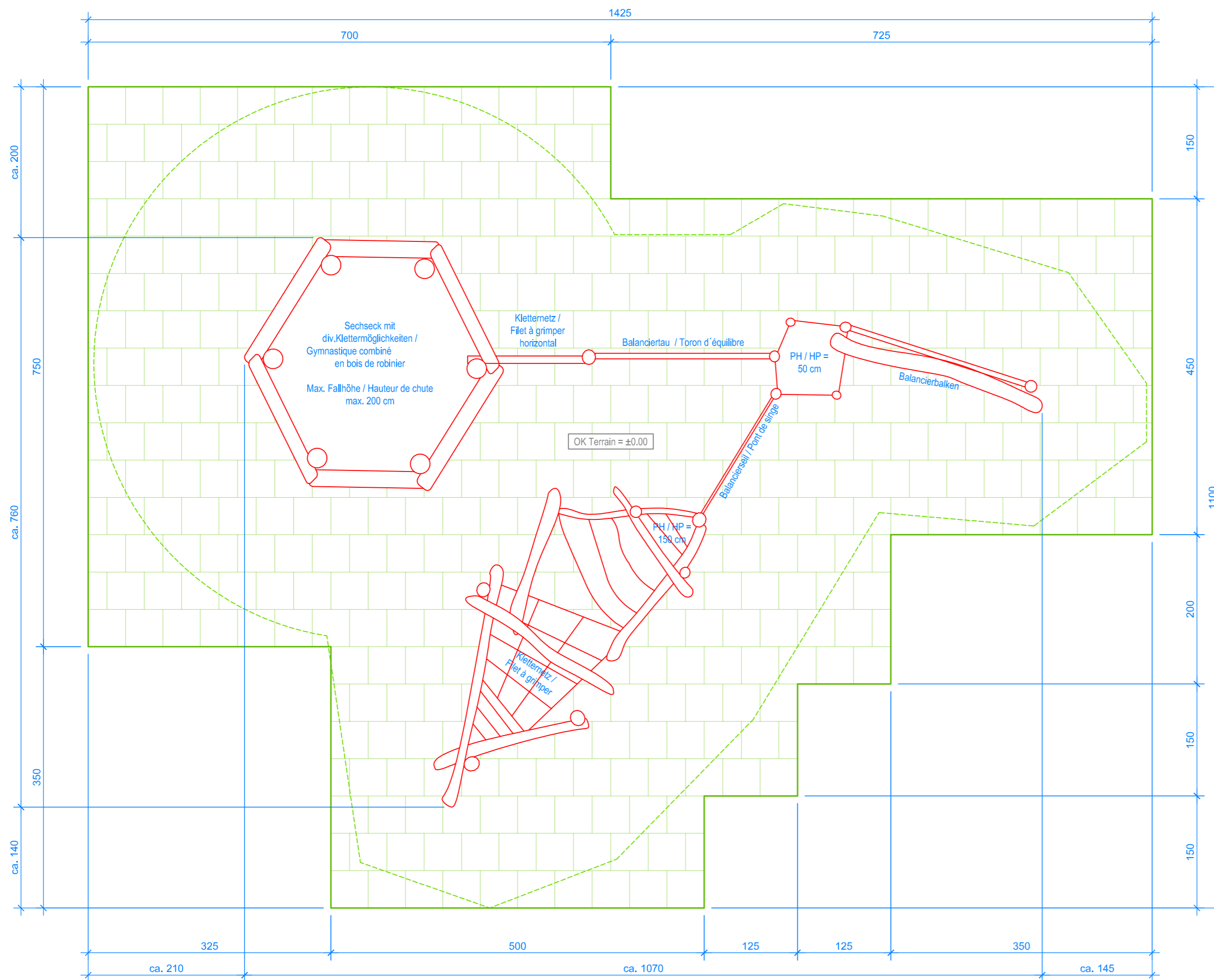
GRUNDRISS / PLAN 1:50
