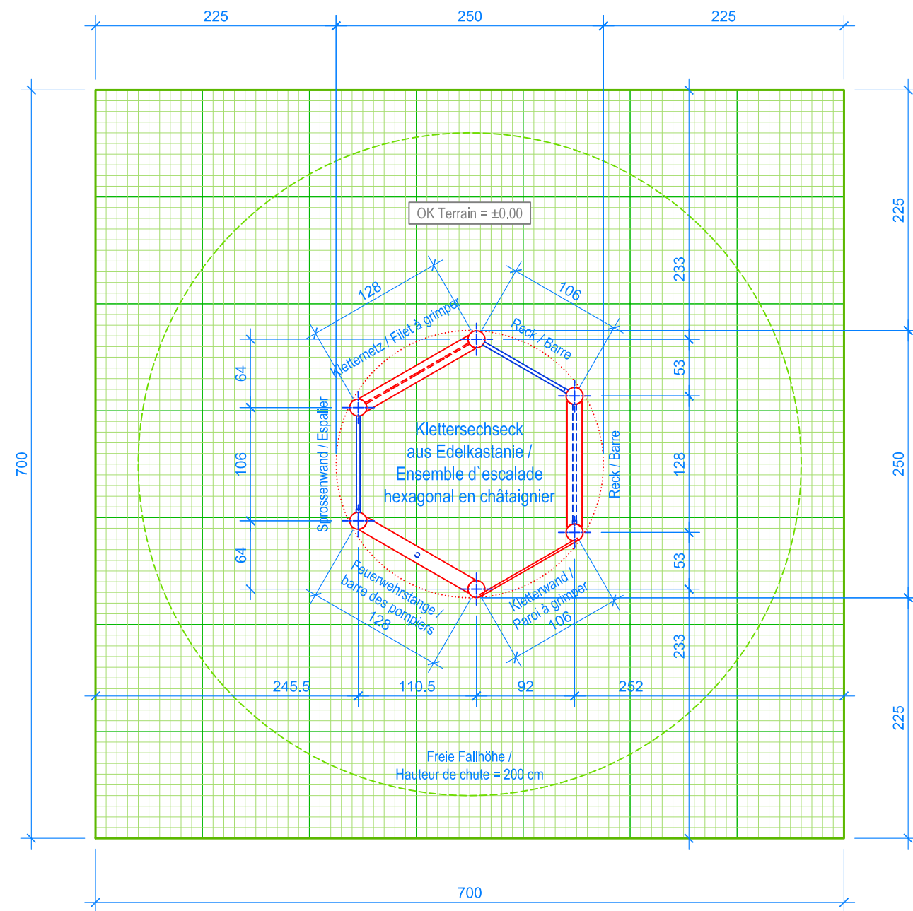
GRUNDRISS / PLAN 1:50
